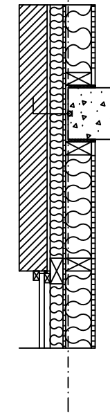
GENERELT HORISONTALSNITT AV YTTERVEGG 1:10
