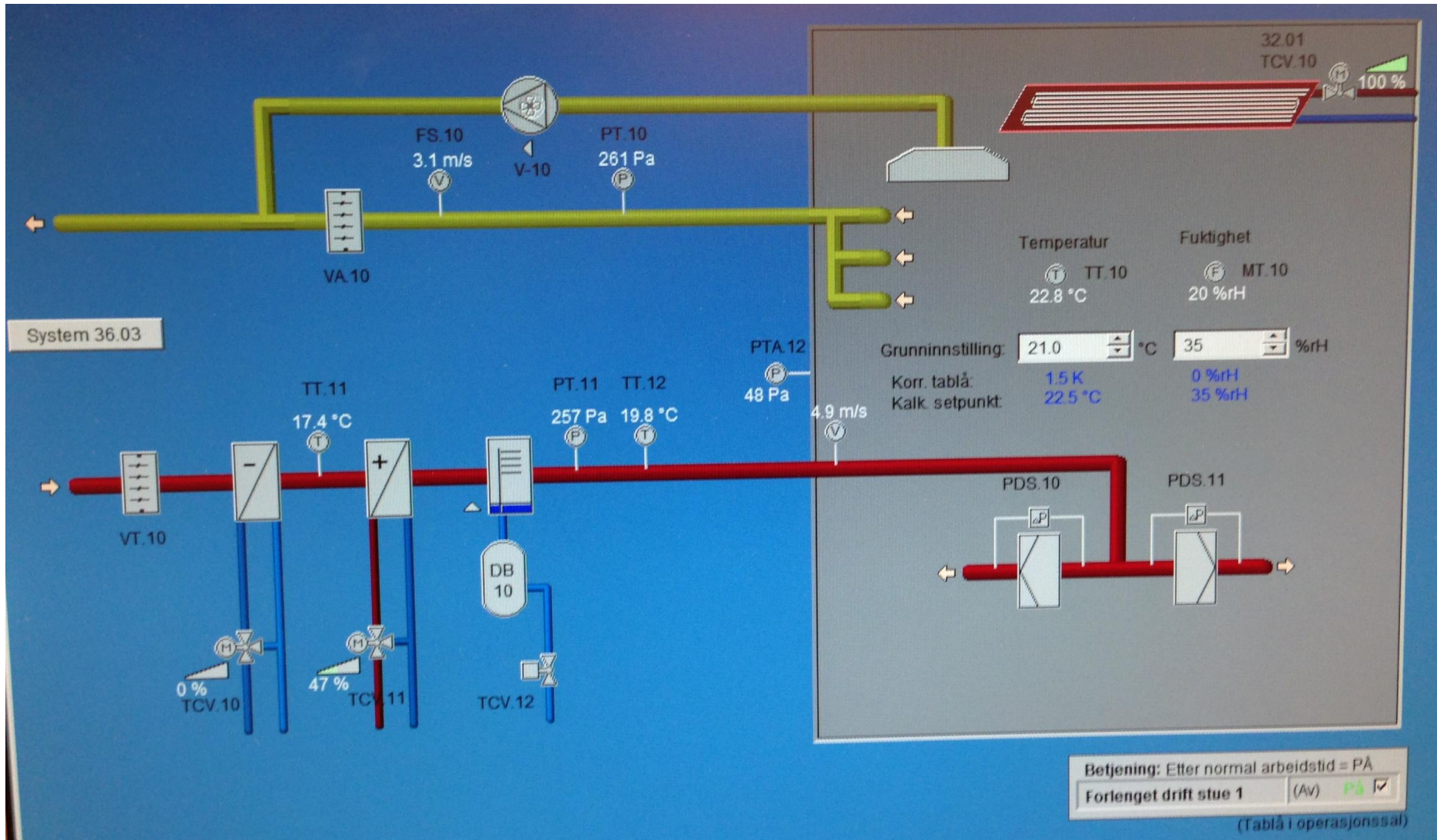
Bilde Desigo Insight system 36.03B OP1:
