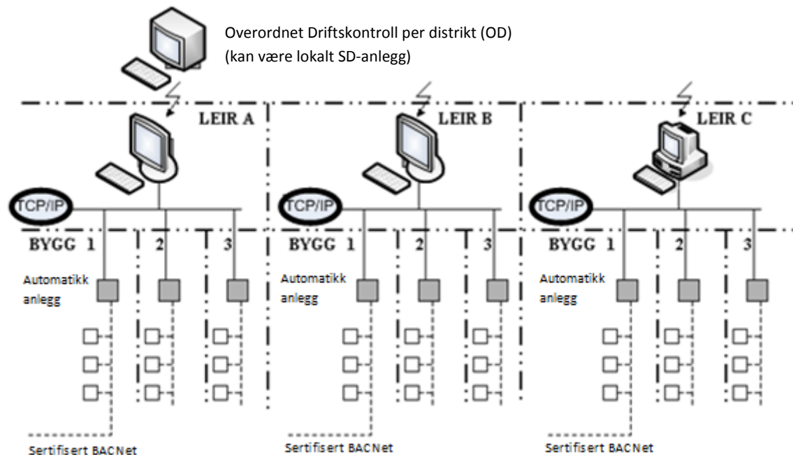
Figur: Prinsipiell nettløsløsning SD-anlegg og automatikkanlegg.
