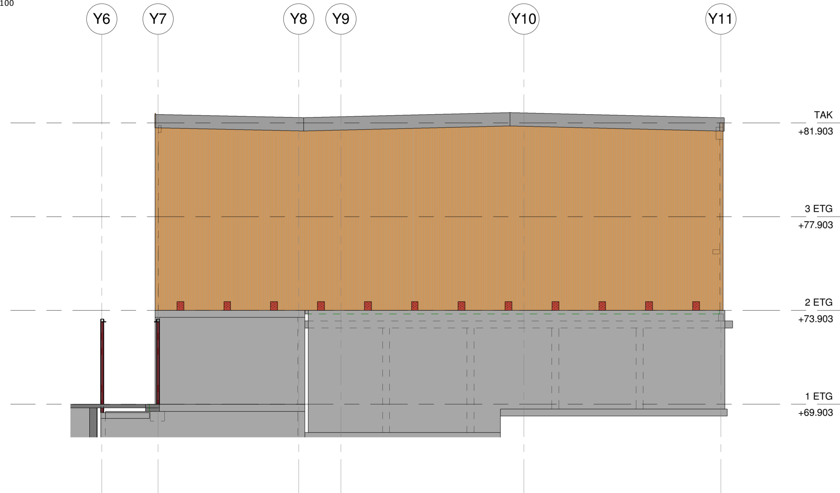
3 Fasade Øst - verksted 1 : 100
