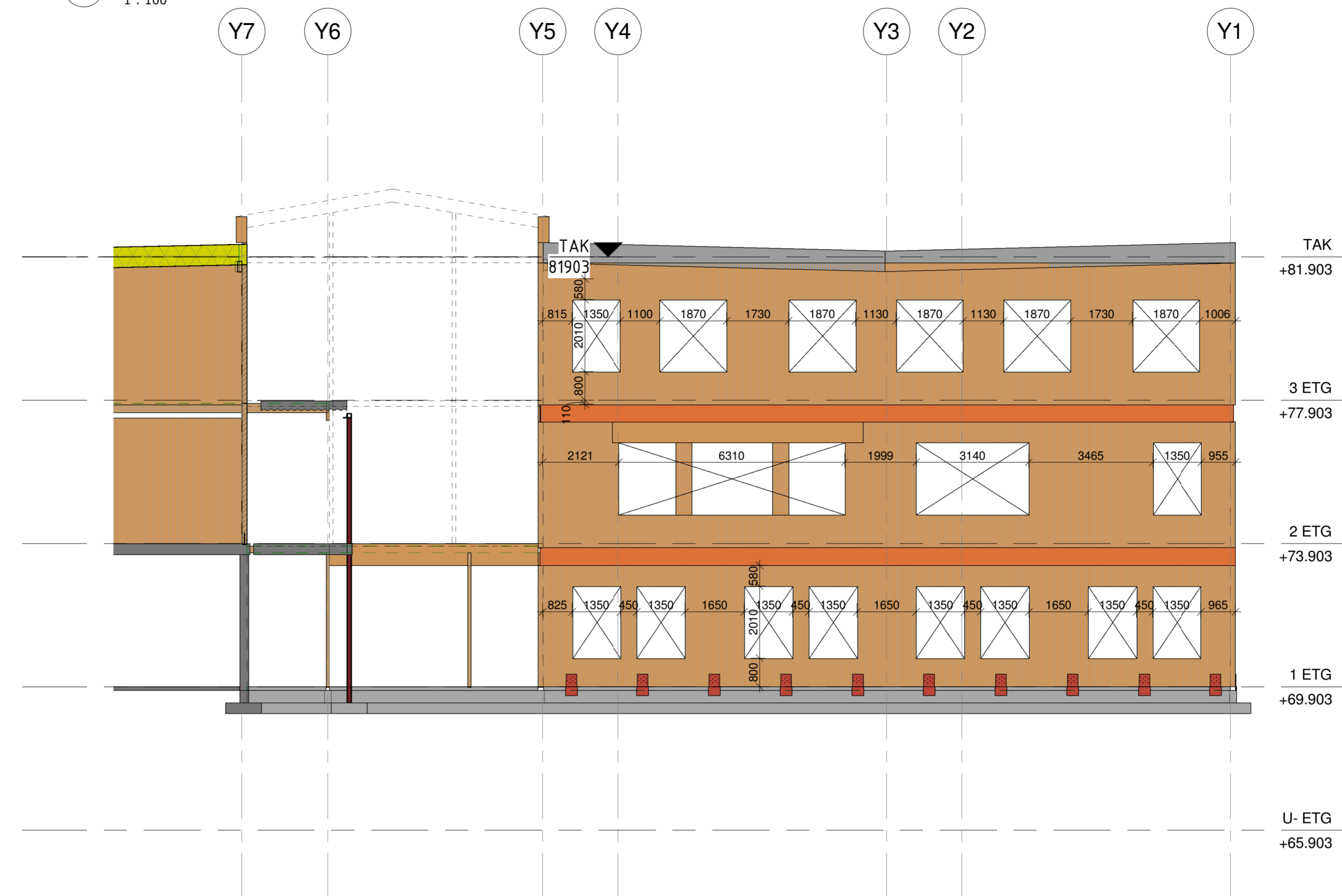
2 Fasade Vest vest fløy 1 : 100
