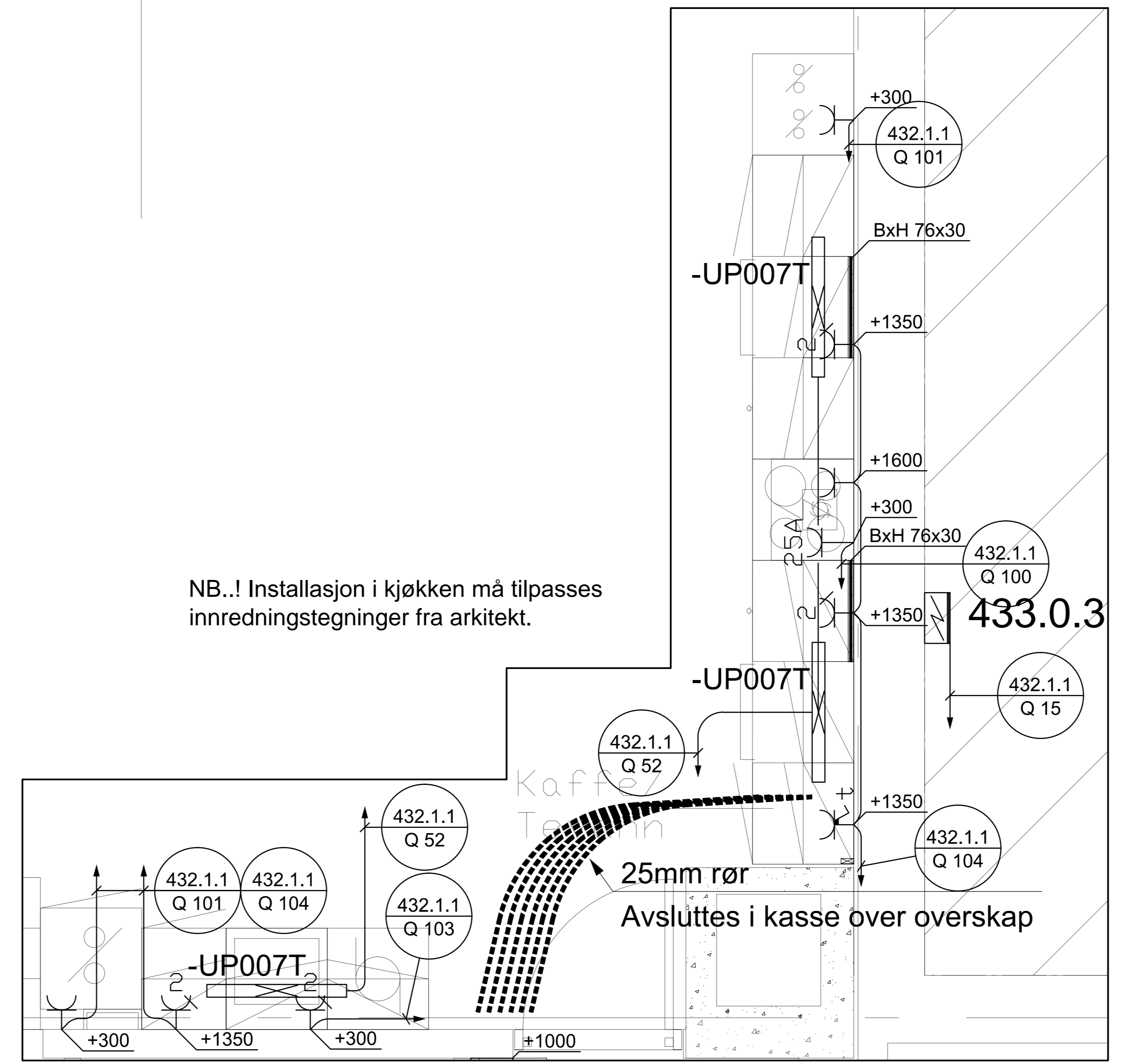
Detalj Kjøkkeninredning 1:20
