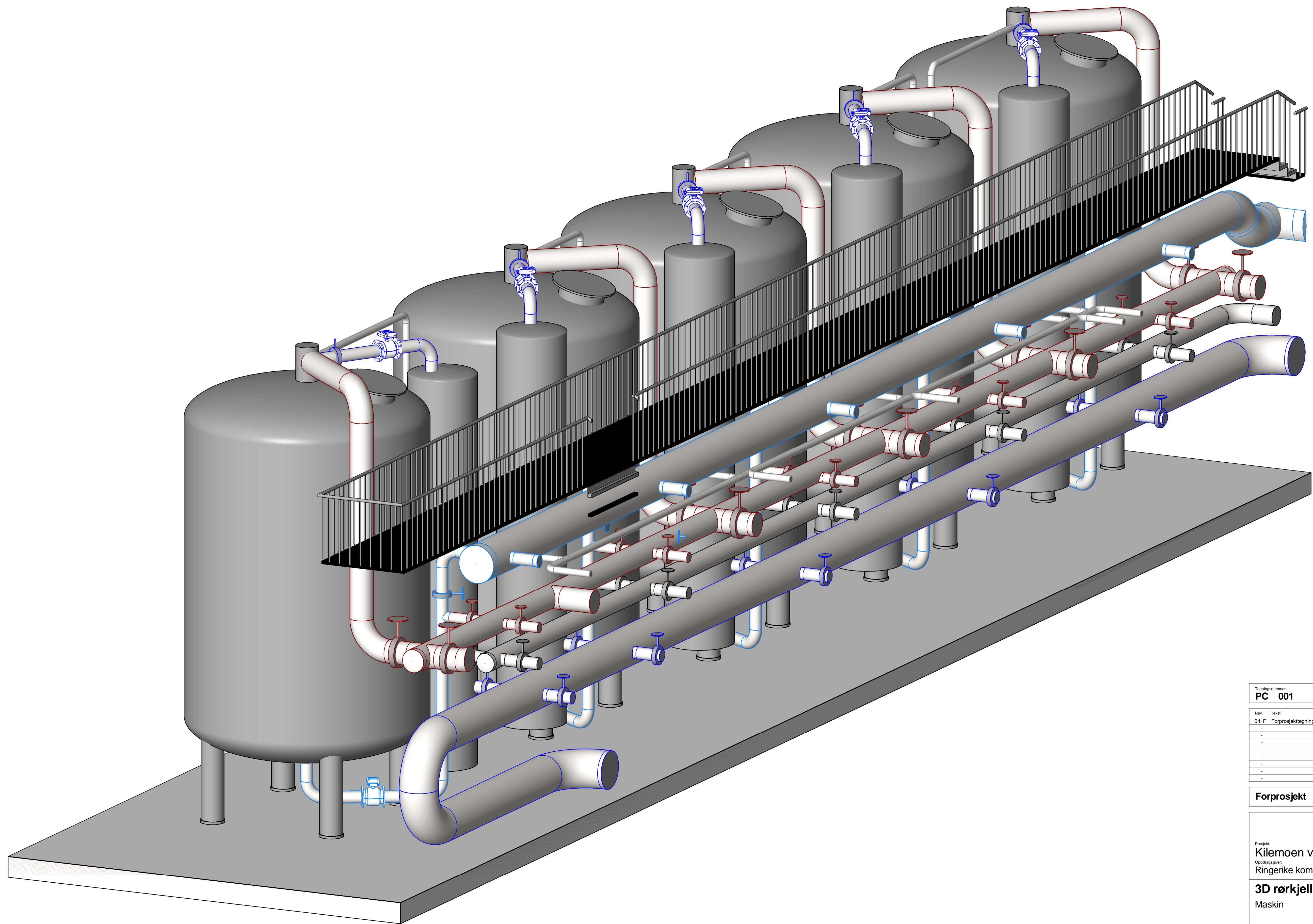
1 3D rørkjeller
