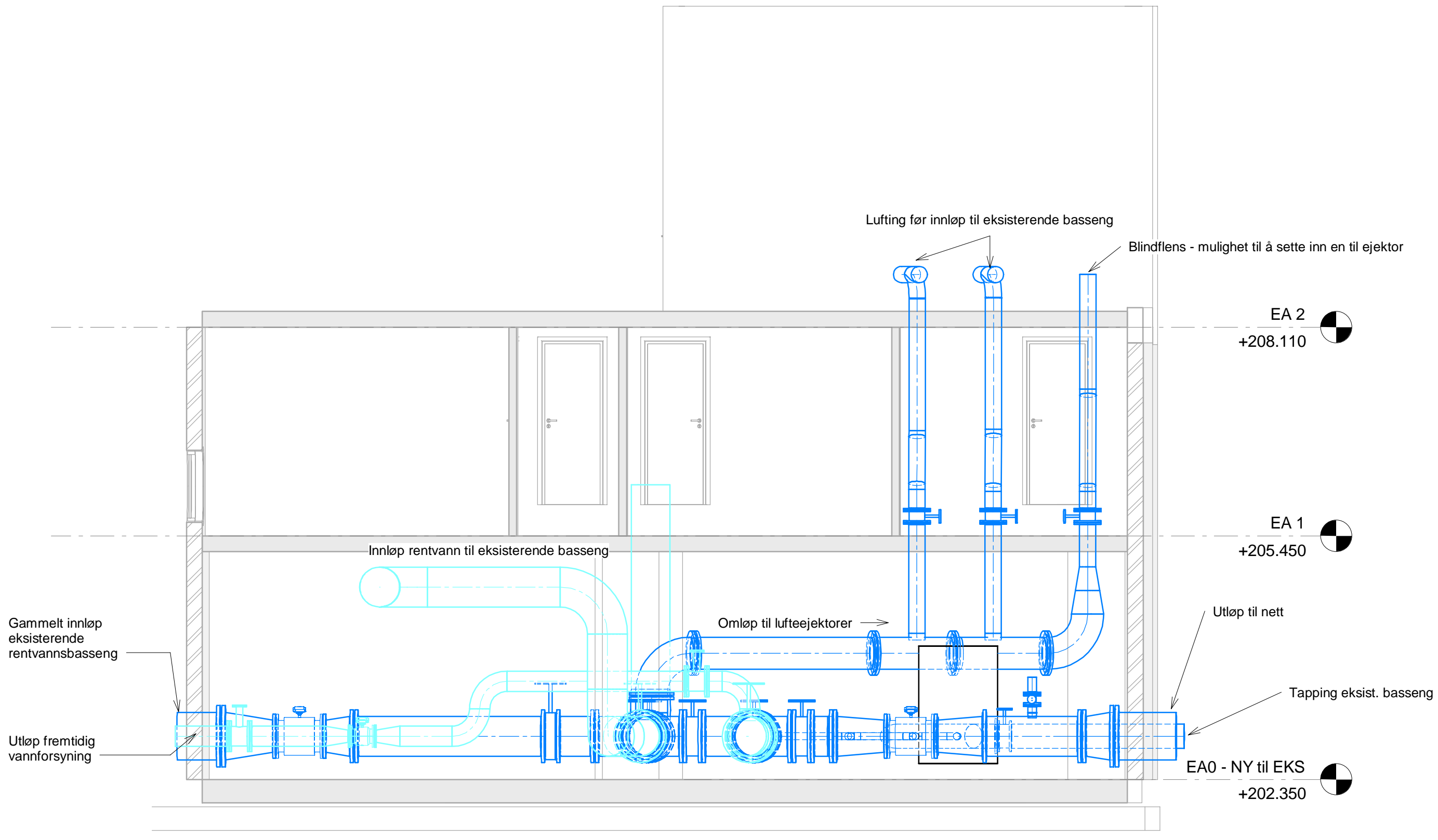
1 Snitt G - ekist. VBA 1 : 50
