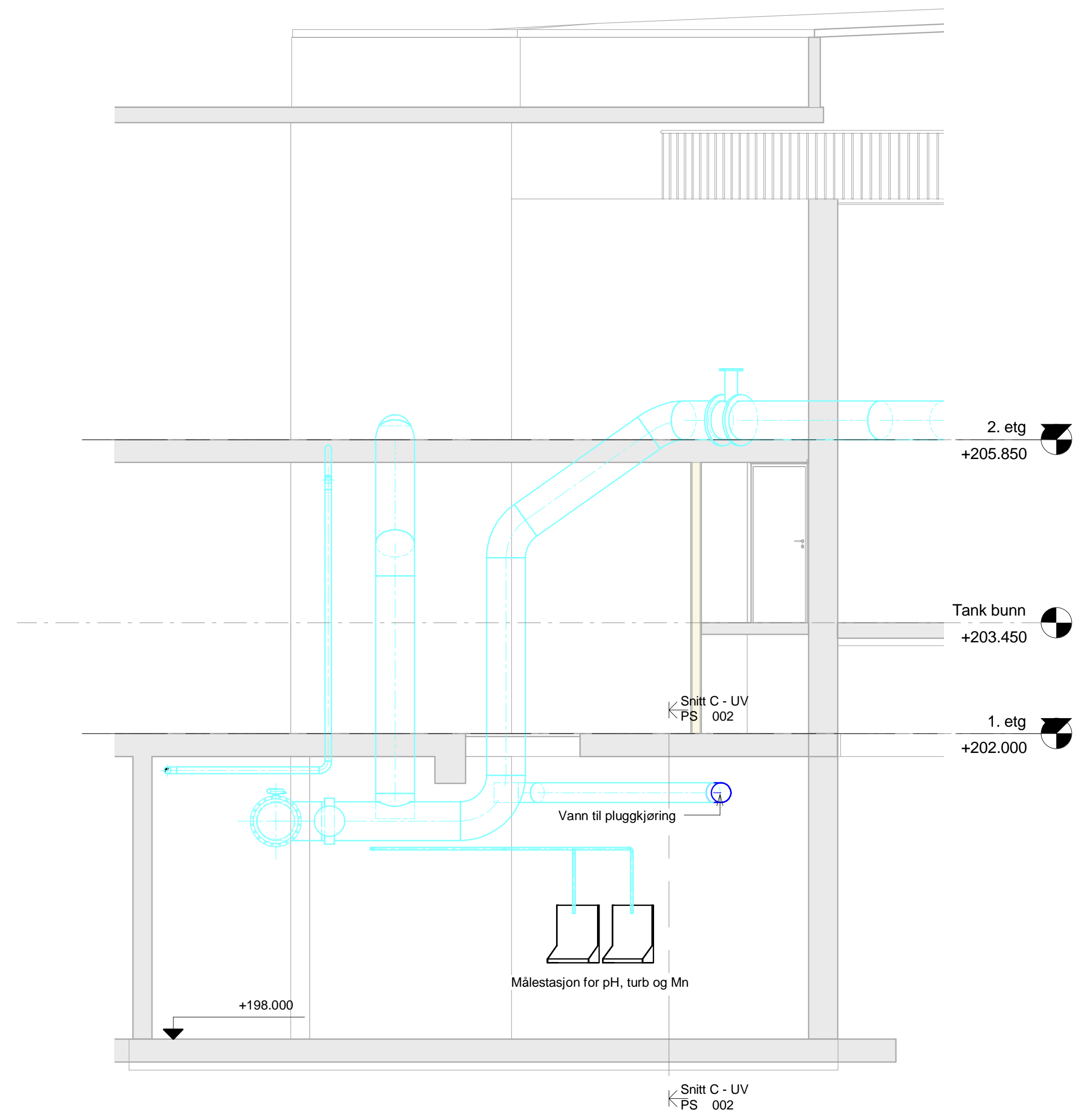
2 Snitt D - Fordeling rentvann 1 : 50
