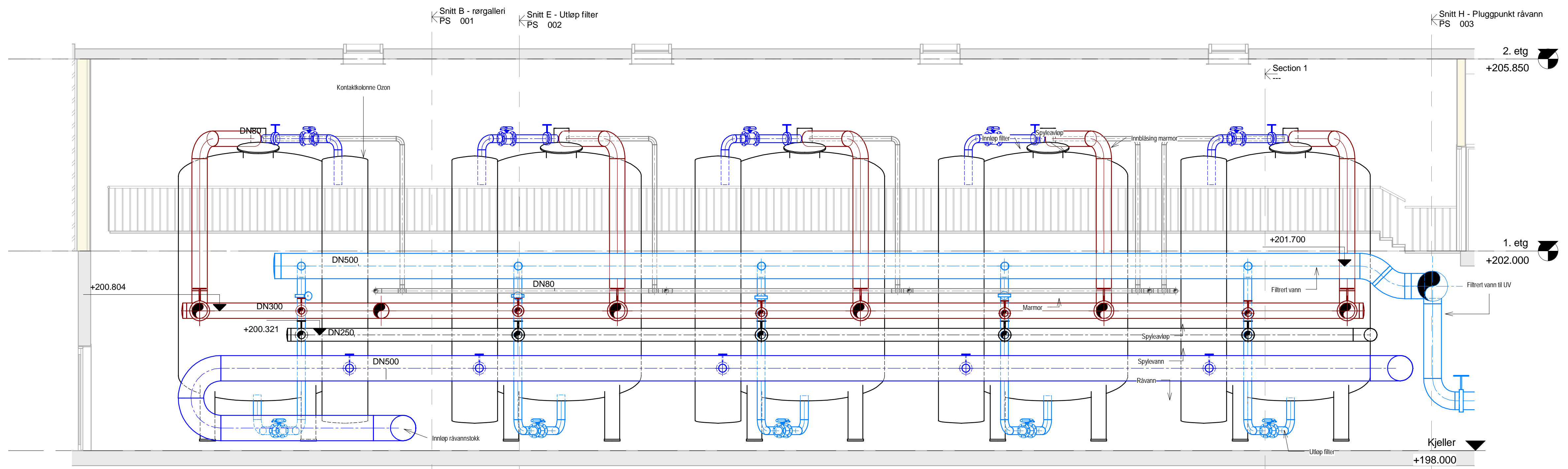
1 Snitt A - rørgalleri 1 : 50
