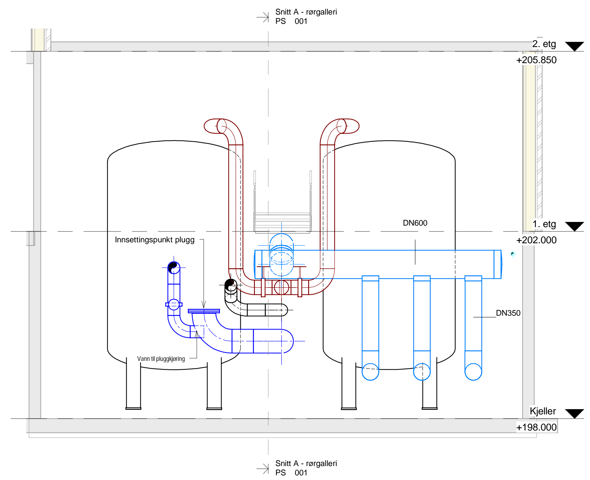
2 Snitt H - Pluggpunkt råvann 1 : 50
