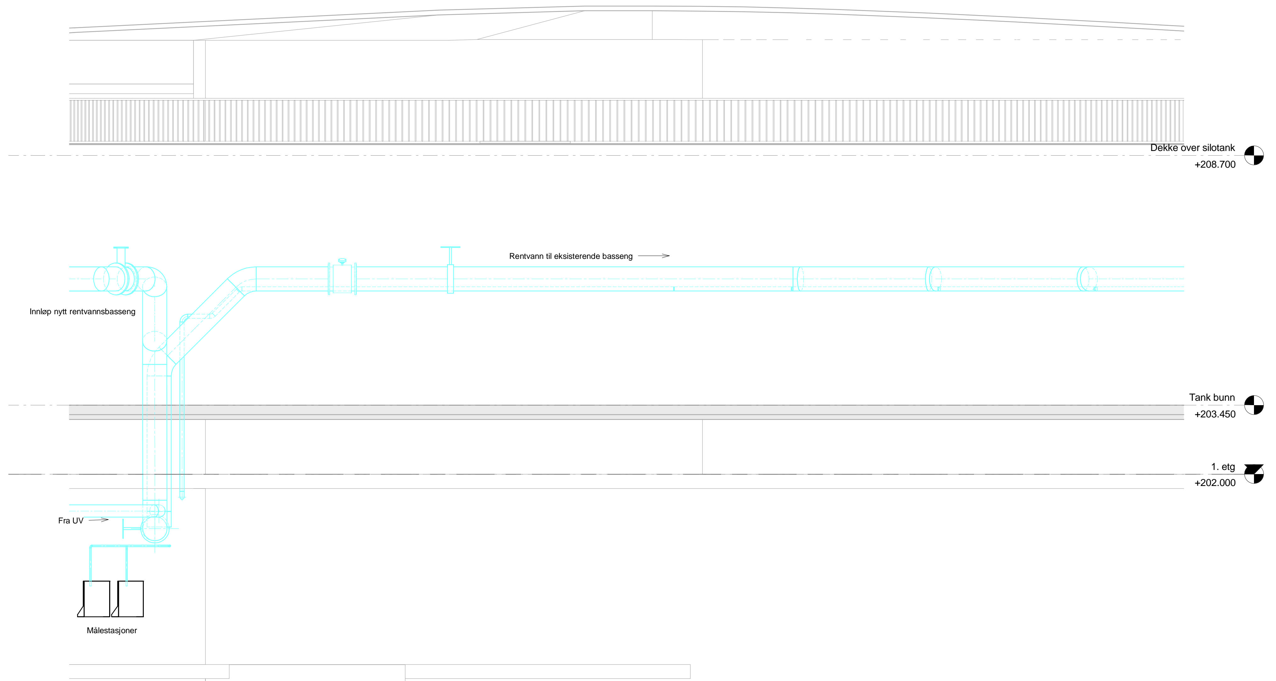
1 Snitt J - fordeling nytt og ekst rentv.basseng 1:50
