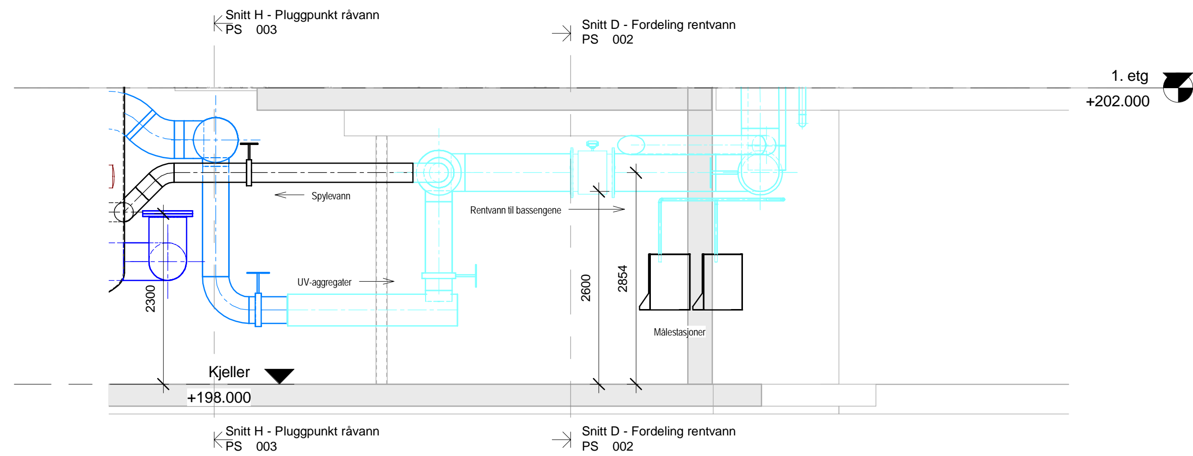
1 Snitt C - UV 1 : 50
