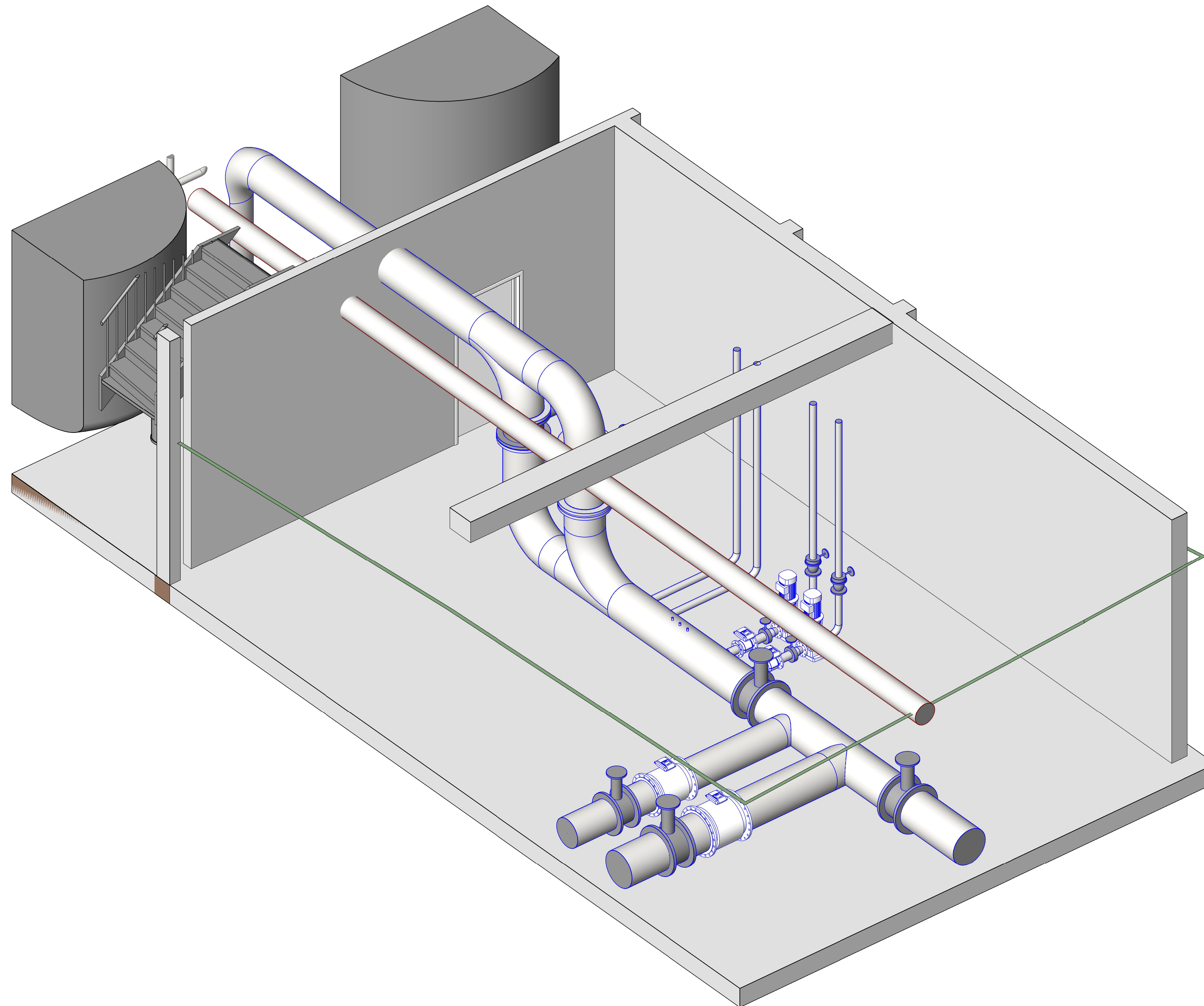
1 3D innløpskjeller
