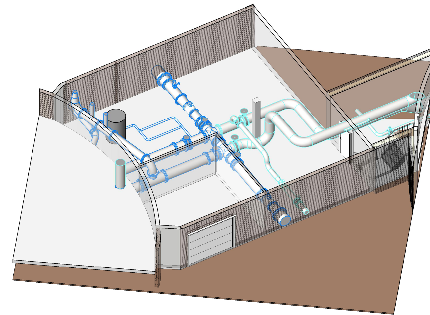
2 3D innløp eksisterende basseng
