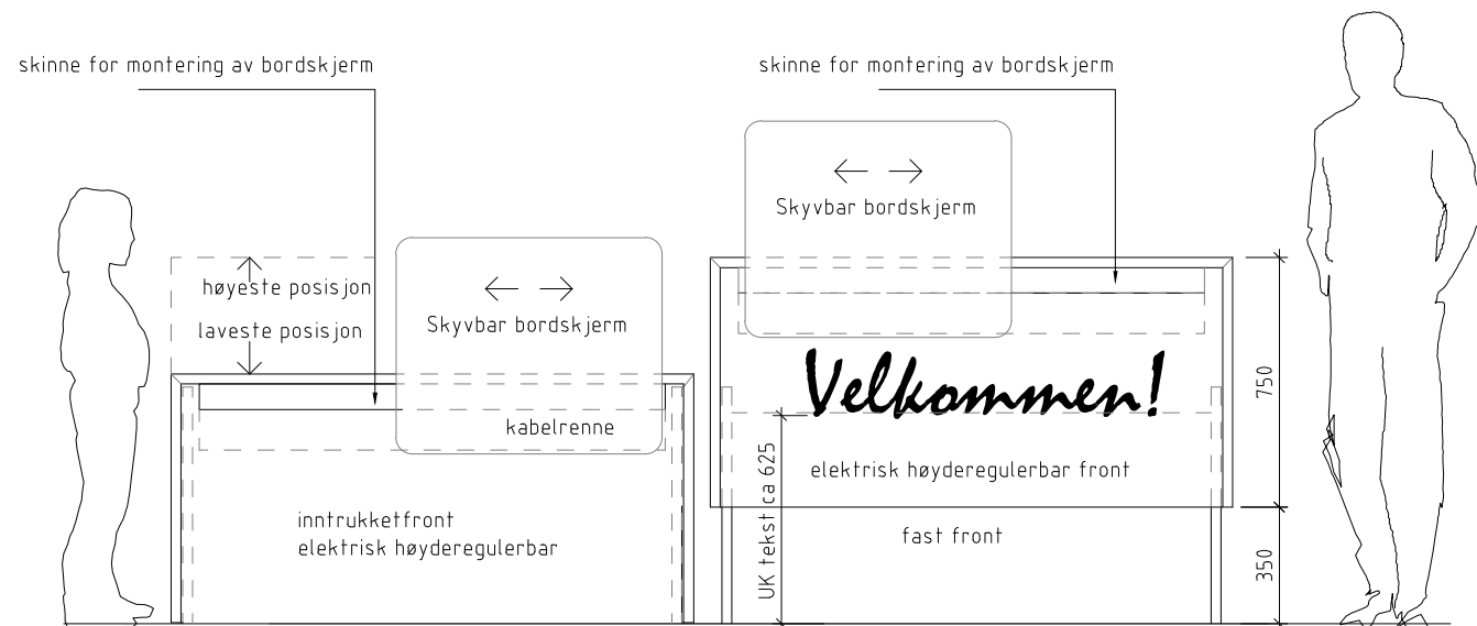
OPPRISS DD, PUBLIKUMSIDE
