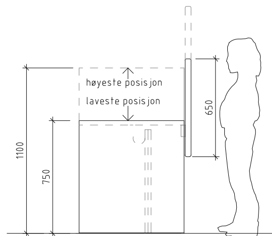
OPPRISS BB, SIDE
