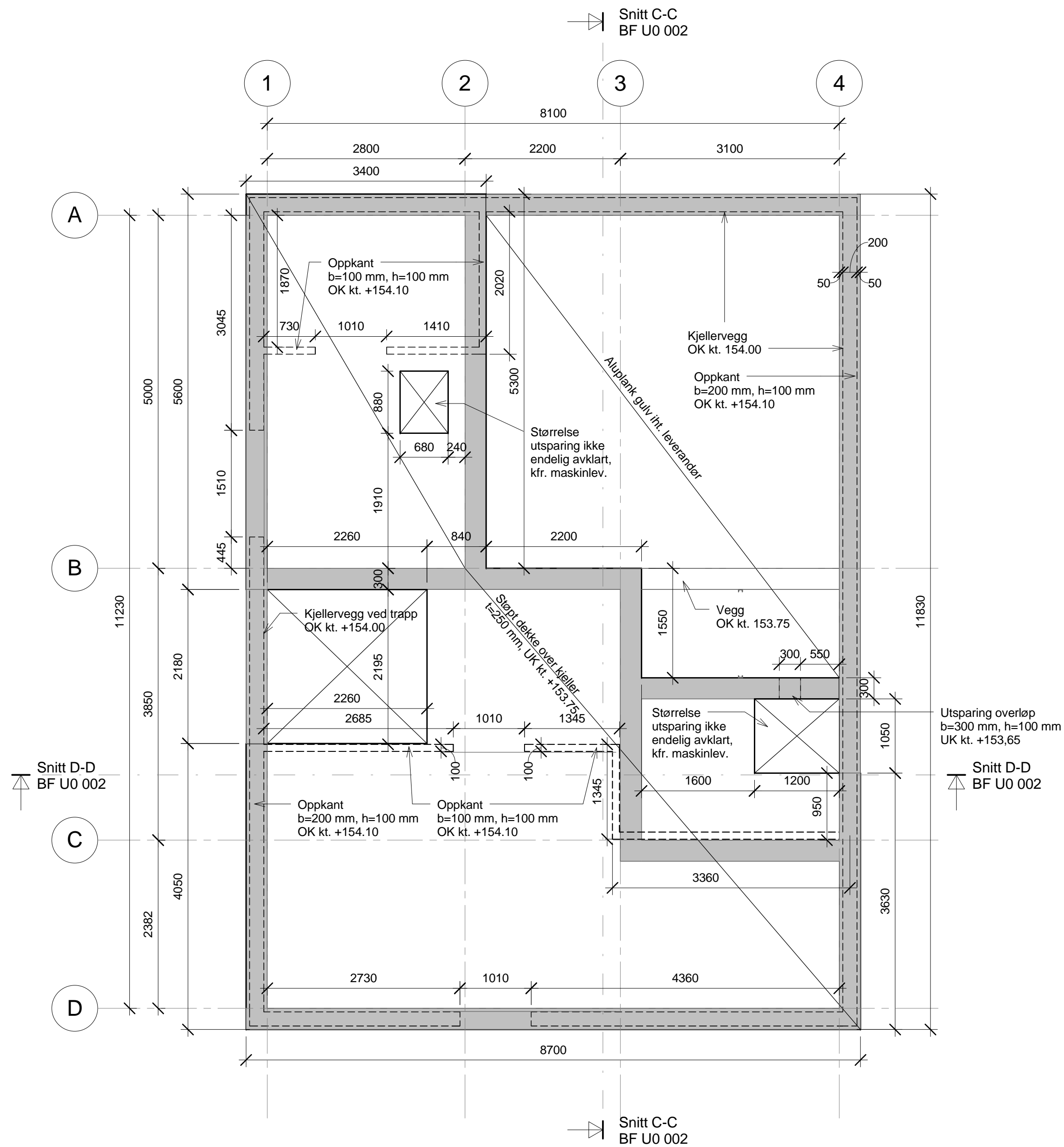
Dekke over kjeller 1 : 50
