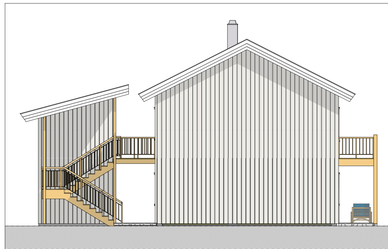
Fasade vest
