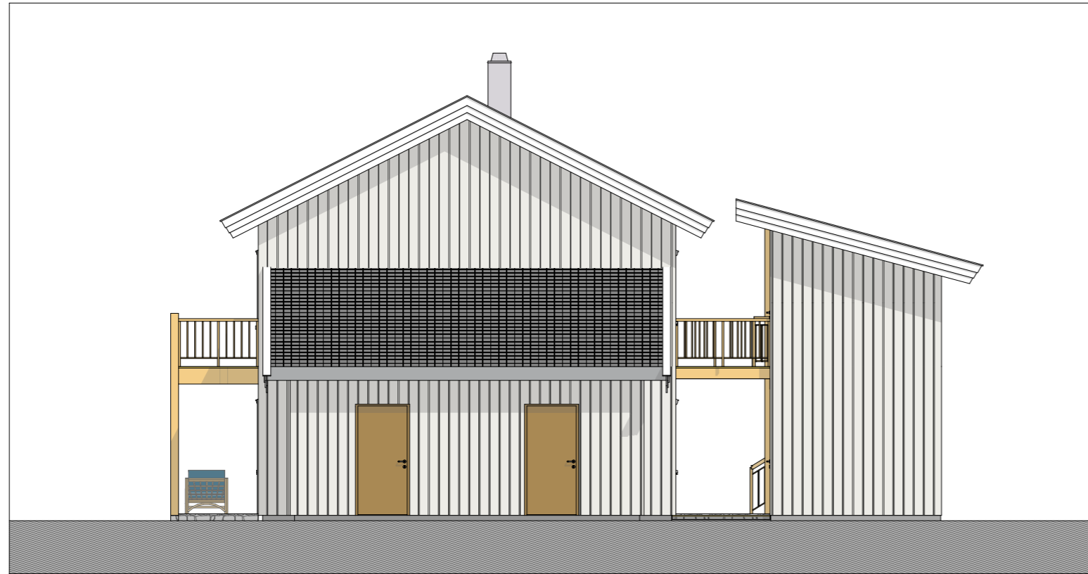
Fasade øst
