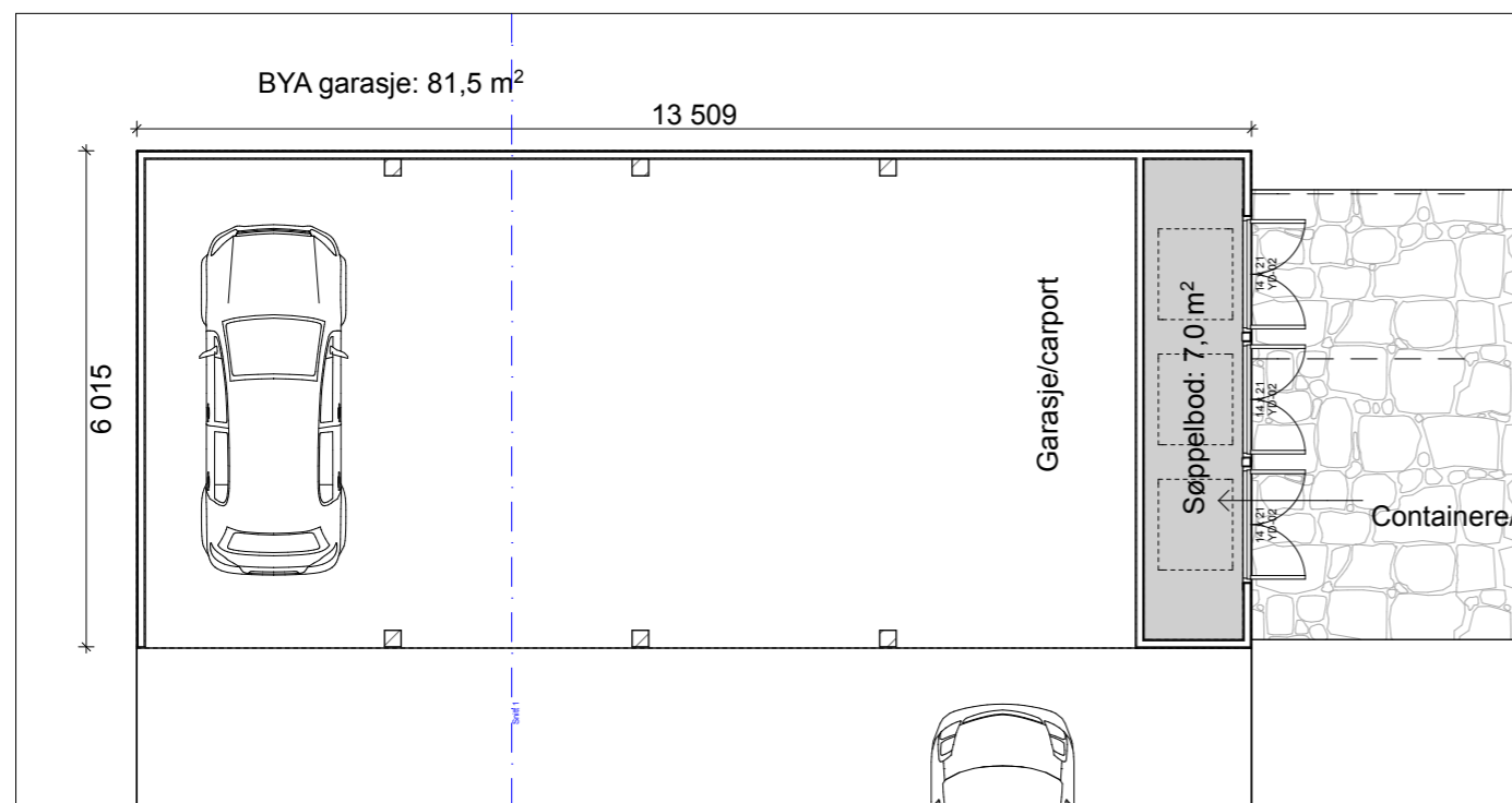
1:100 Plan
