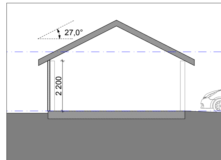
1:100 Plan
