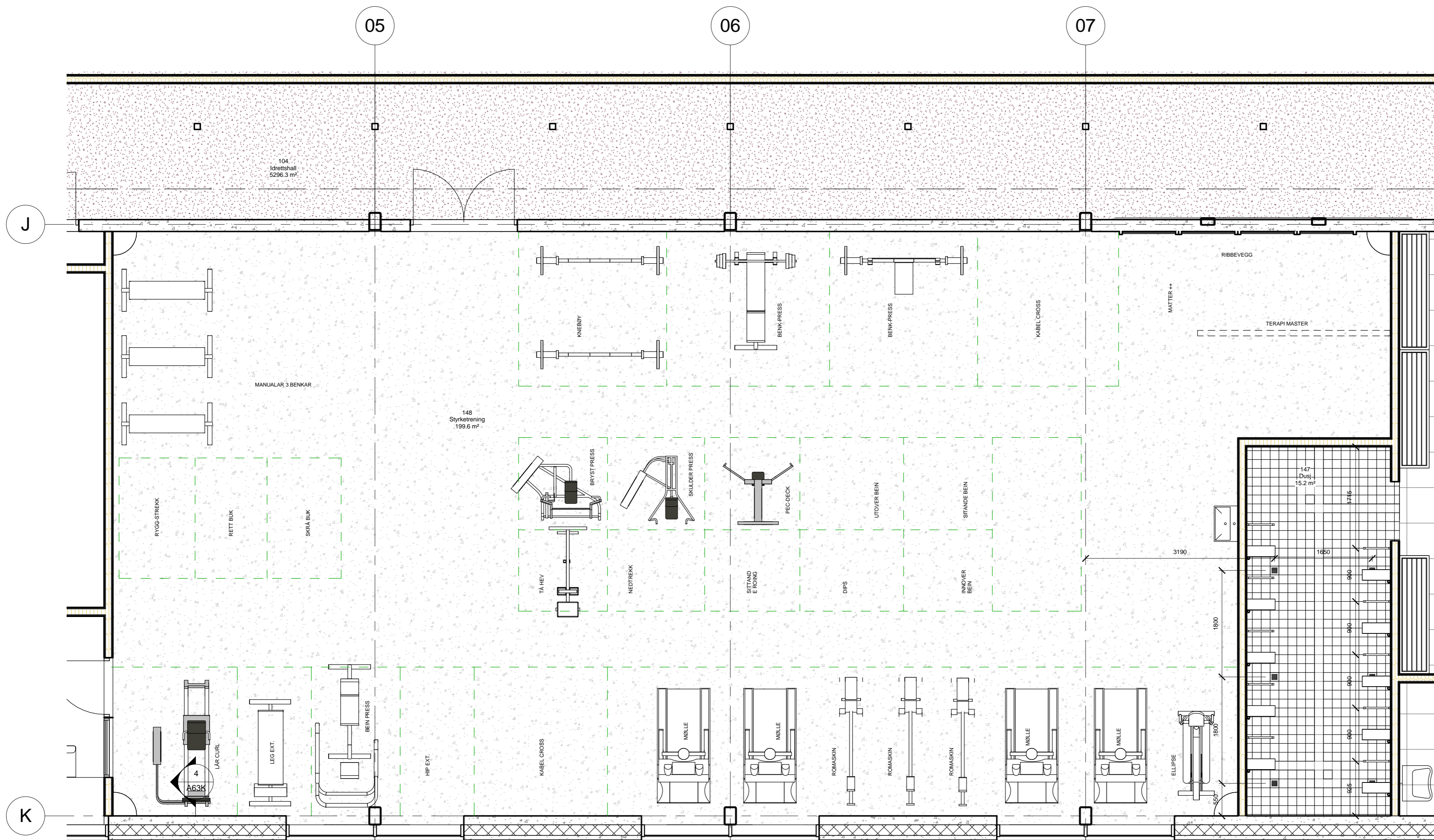
1 Plan styrkerom 1:50
