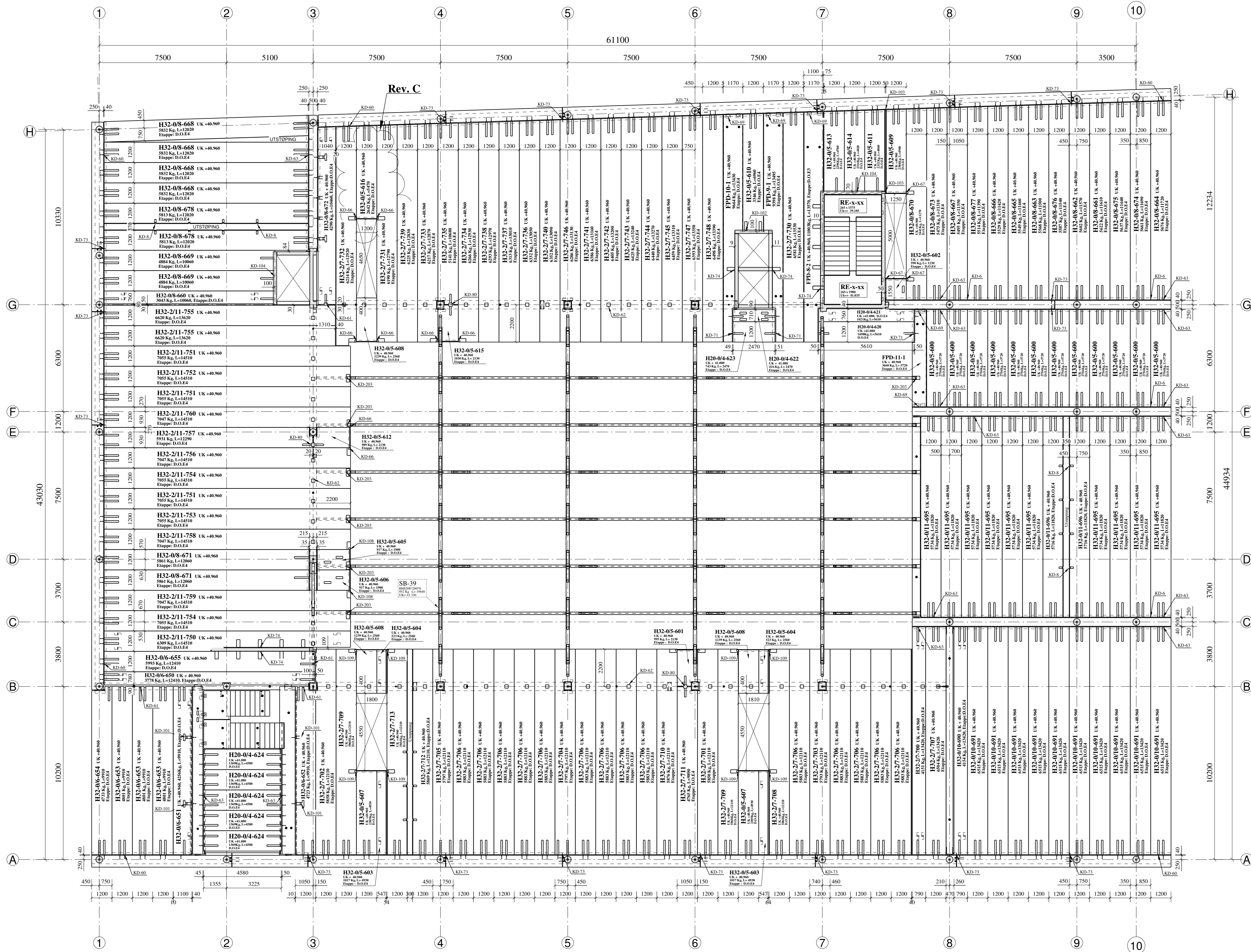
PLAN +40.960 (E4 og d.o.) 1:100
