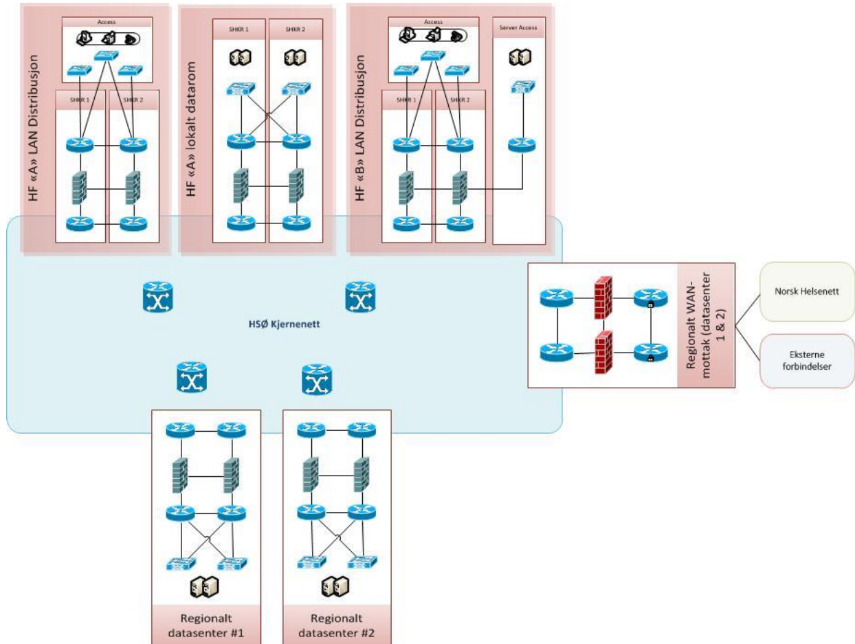
Figur 8.1 – 2 Overordnet nettverksdesign
