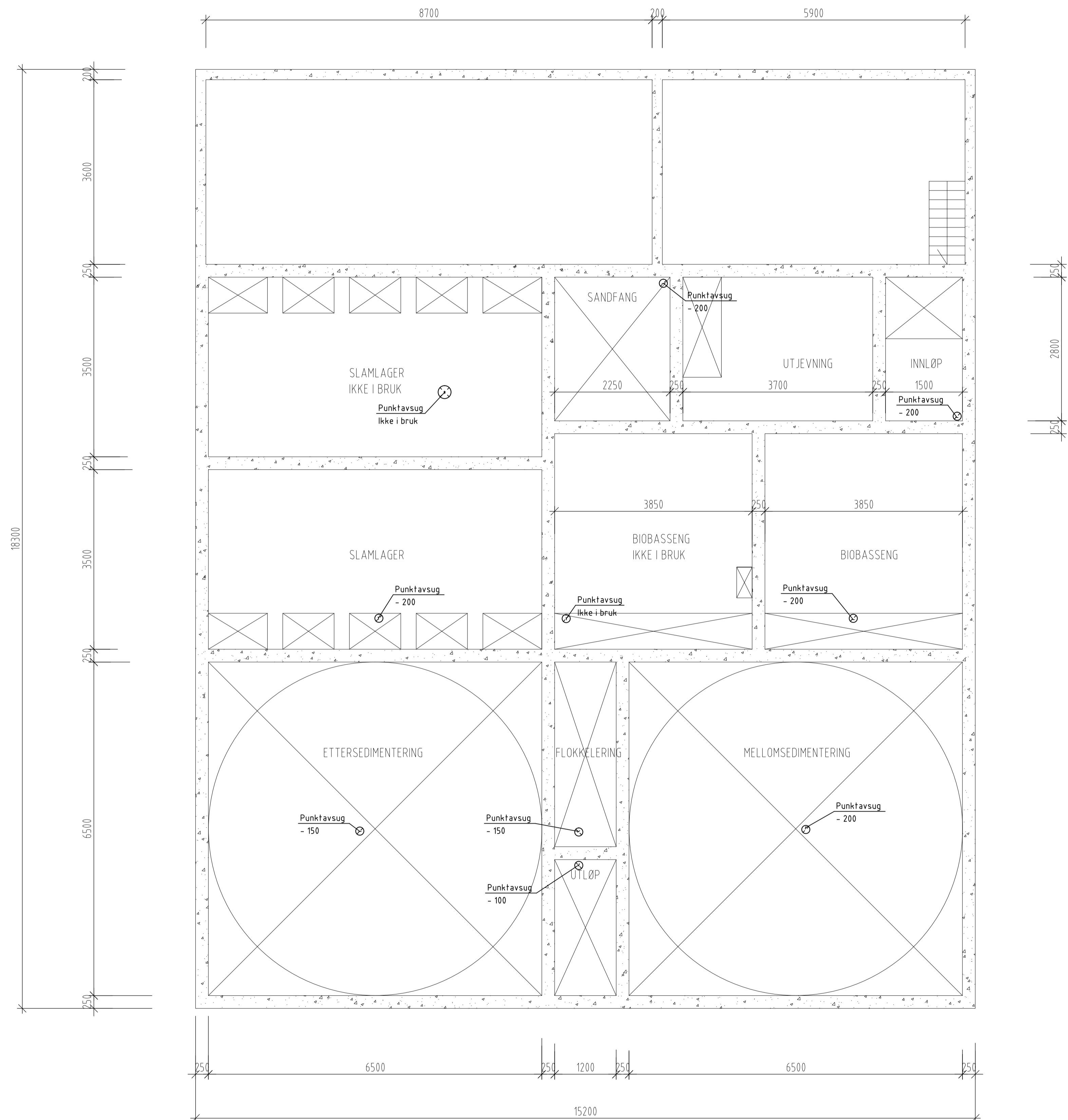
PLAN U 1:50
