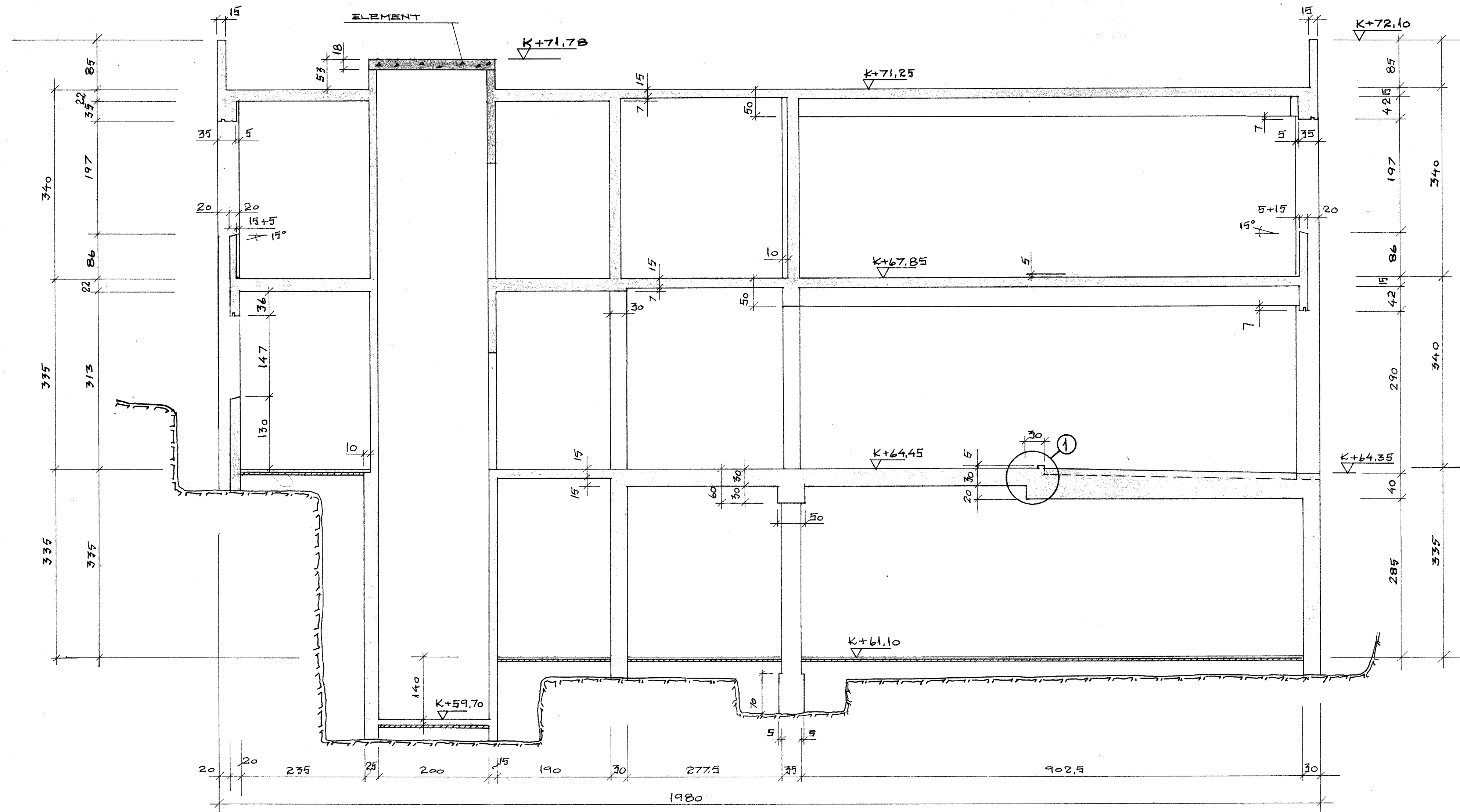
SNITT A-A 1:50
