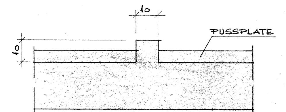
SOKKEL FOR MURSTEINVEGG 1:10 PÅ GOLV OVER KJELLER/1. ETASJE
