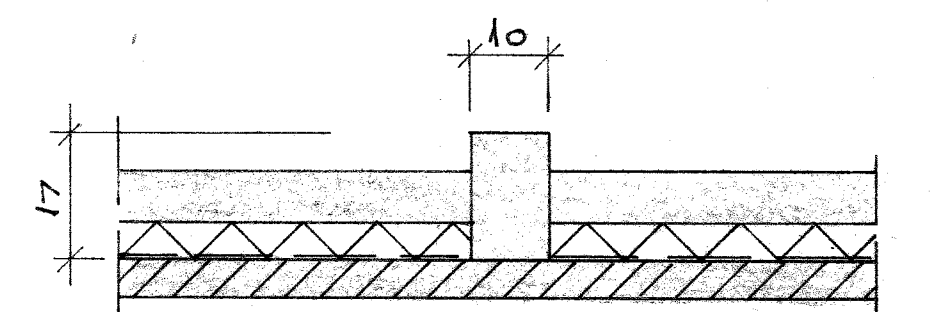
SOKKEL FOR MURSTEINVEGG 1:10 PLATE PÅ MARK
