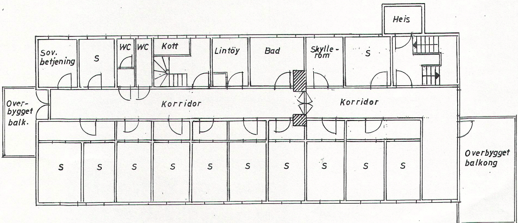
TYRIBO 2. ETASJE M. 1:200 -87
