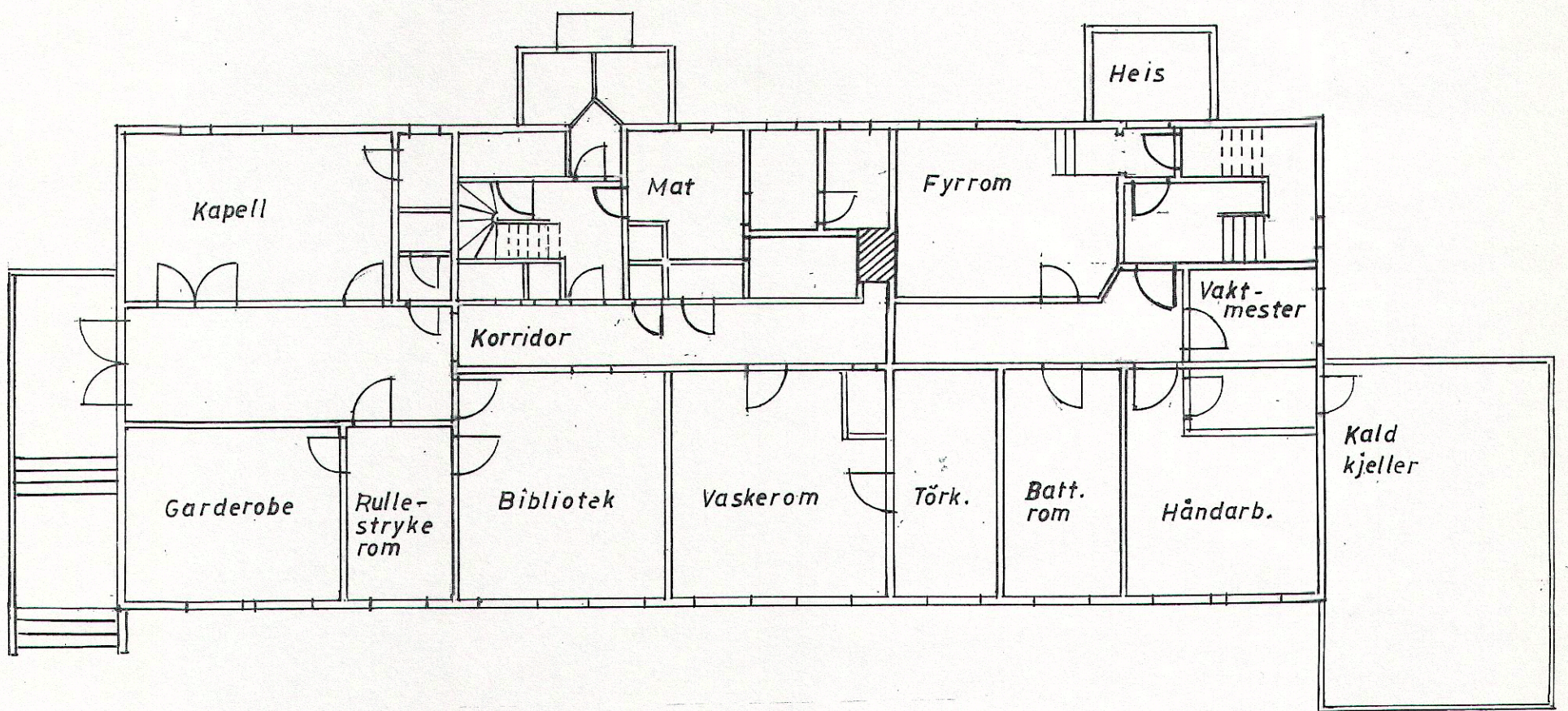
TYRIBO KJELLER M. 1:200 -87
