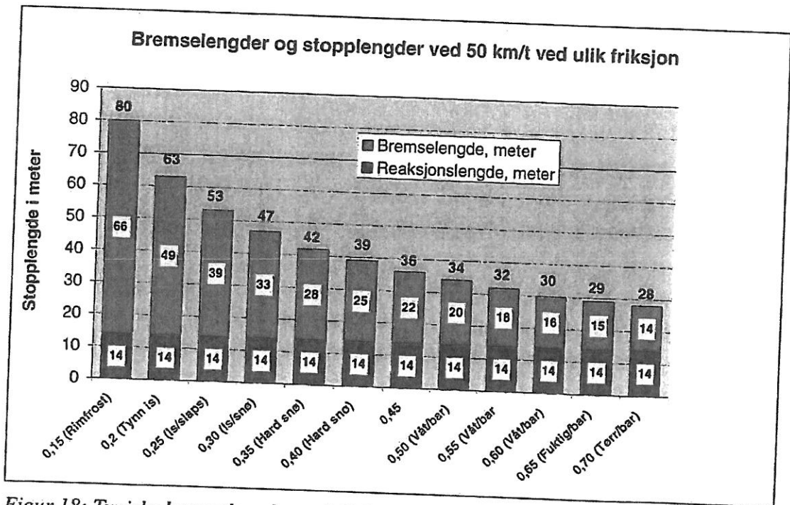
Figur 18: Typiske bremselengder ved 50 km/t ved ulike friksjon
