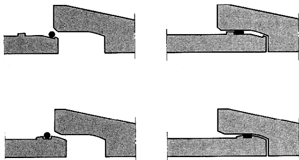
Figur 1: Figuren viser fleksible skjøter, øverst rullepakning og nederst glidepakning.
