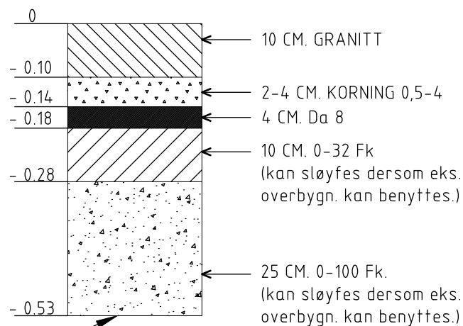
OVERBYGNING FORTAU MED NATURSTEINSBELEGG 1:10
