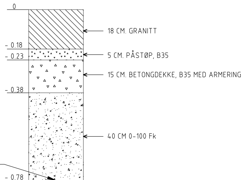
OVERBYGNING KJØREAREAL MED NATURSTEINSBELEGG 1:10
