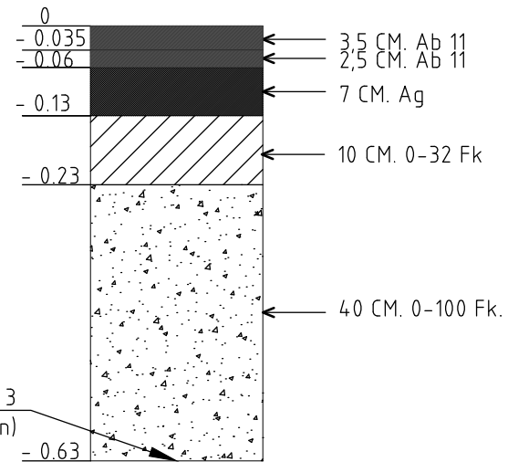
OVERBYGNING GATE MED ASFALTDEKKE TOLLEF KILDES GATE (sør for Torggata) OG FV 215 1:10
