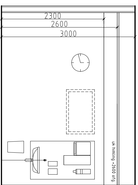
OPPRISS A-A
