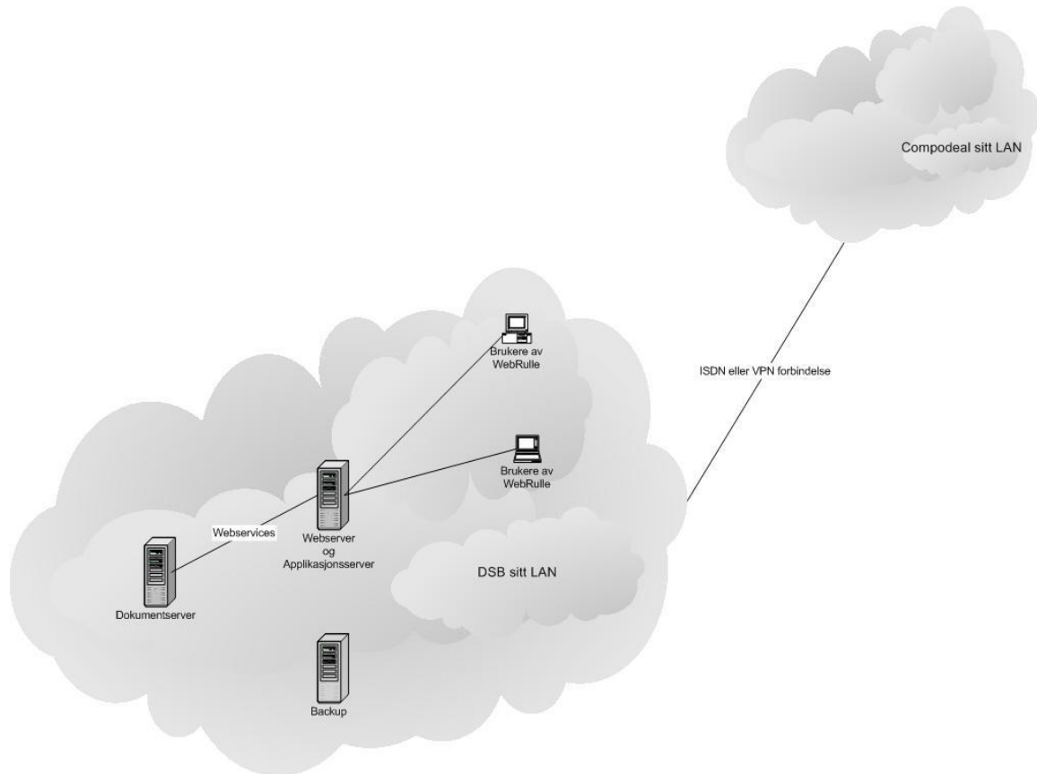
Figure 2 Fysisk skisse.
