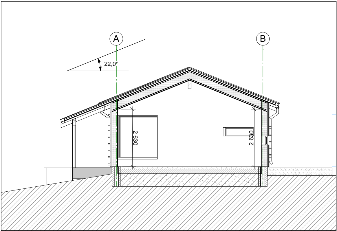
S-4 Snitt akse 7-8+ 1:100
