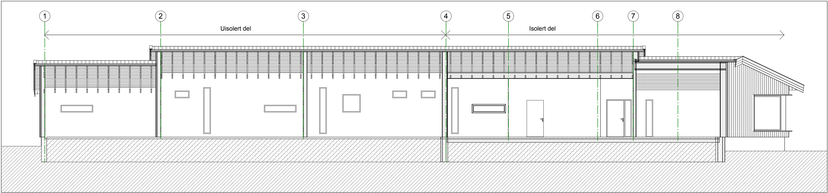
LS-1 Snitt 1:100
