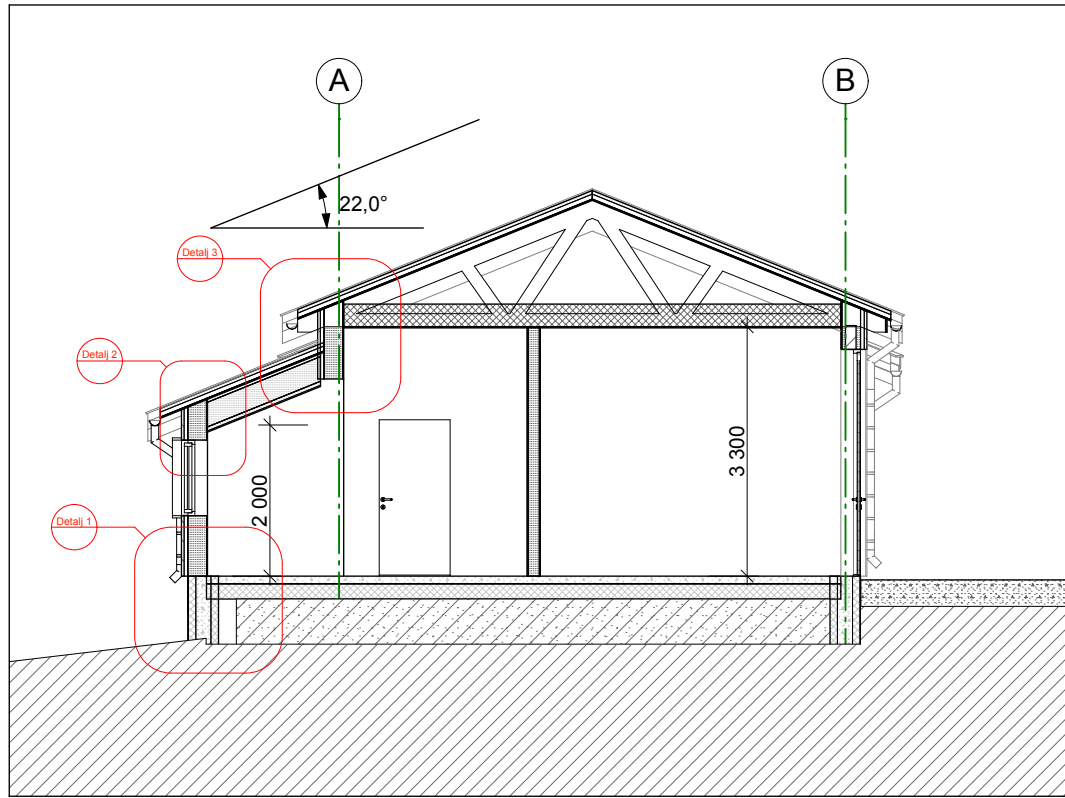
S-3 Snitt akse 4-7 1:100
