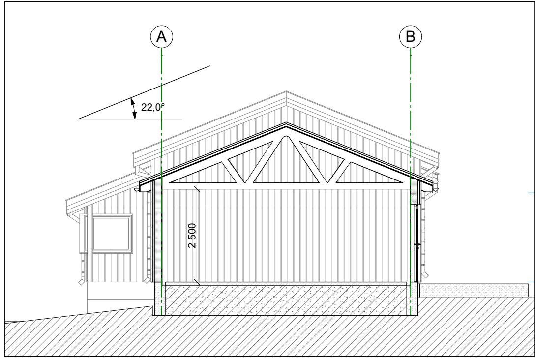
S-1 Snitt akse 1-2 1:100
