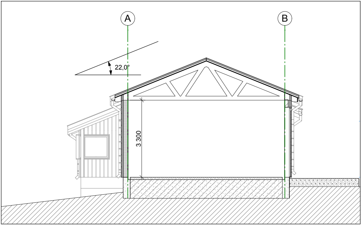
S-2 Snitt akse 2-4 1:100
