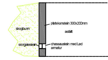
PLAN 1:100 Ledelinjer i granitt med Ledbelysning i Chassastein
