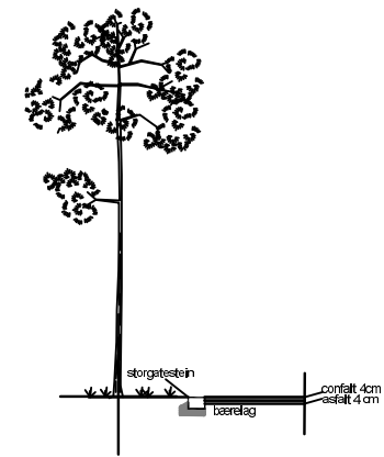
SNITT 1:100 Kanting av skatebane med confalt
