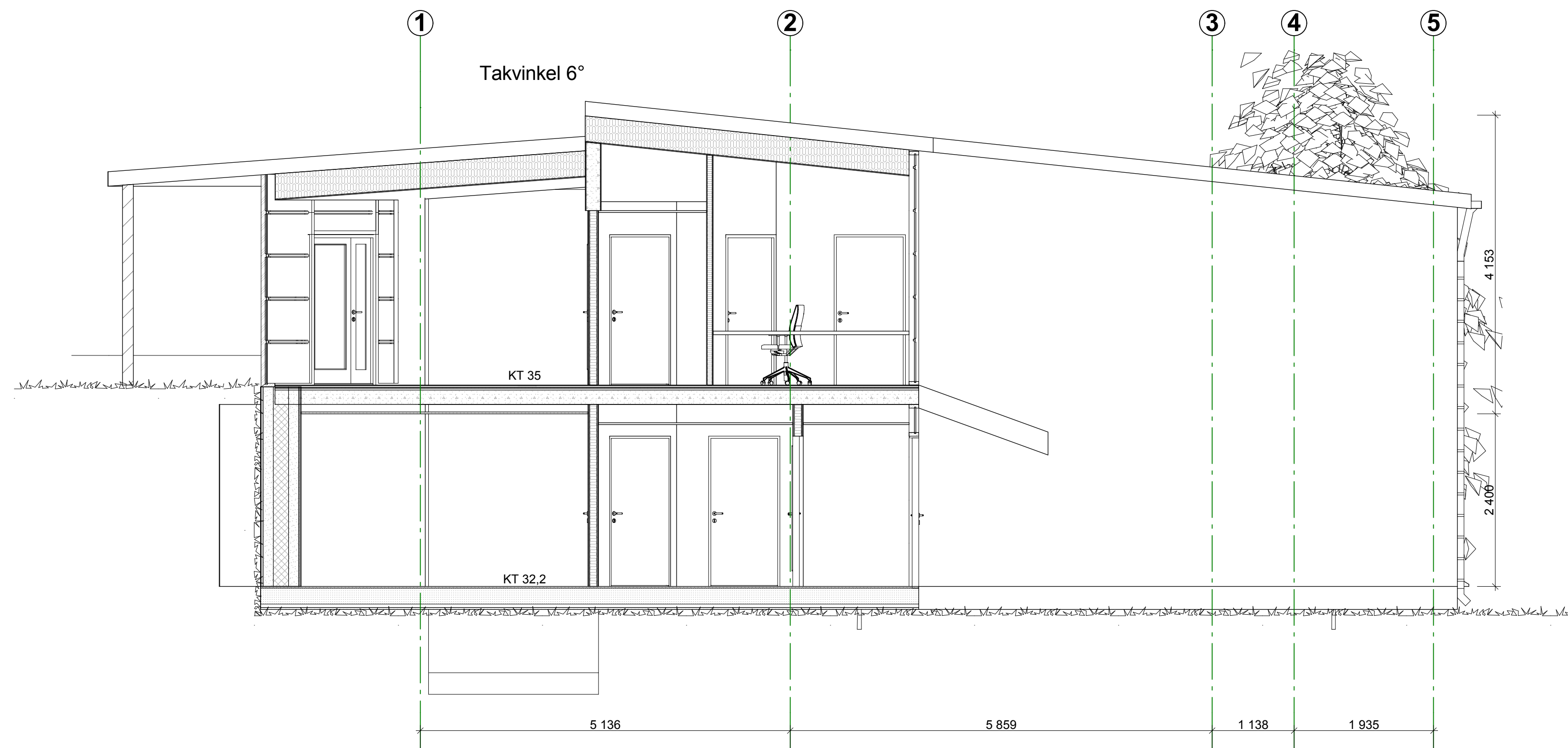
Snitt AA 1:50
