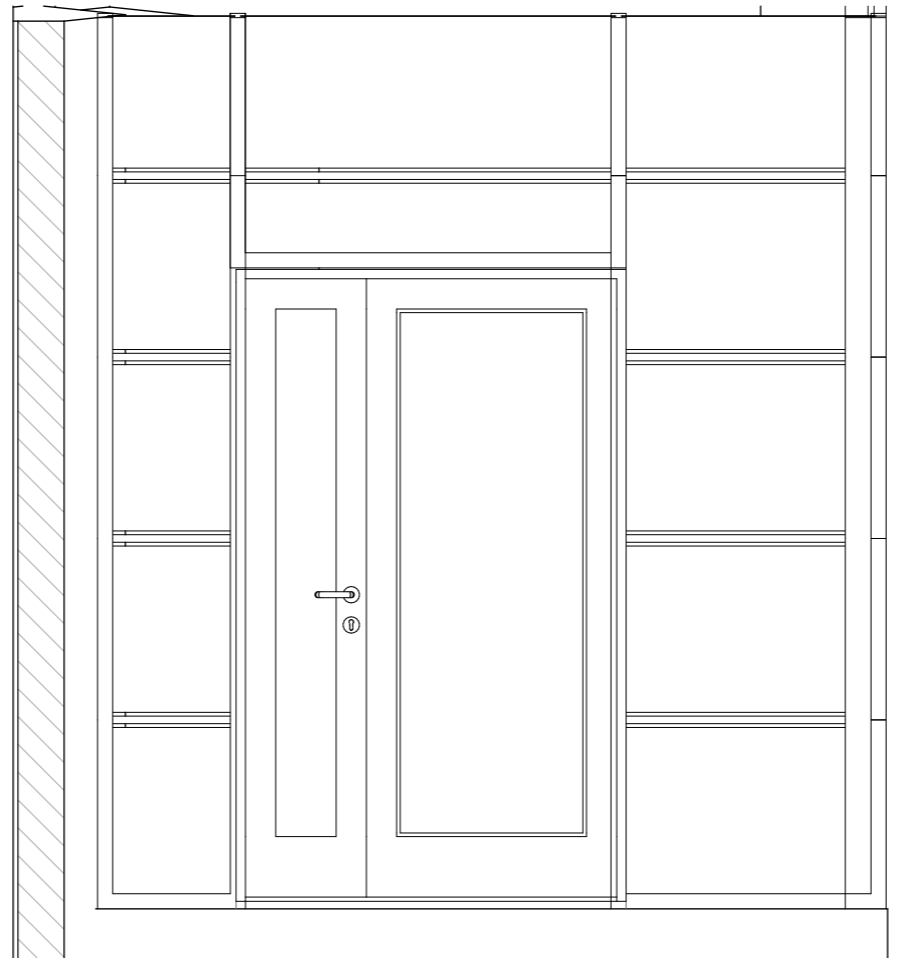
Oppriss nord-øst mot hovedinngang 1:25
