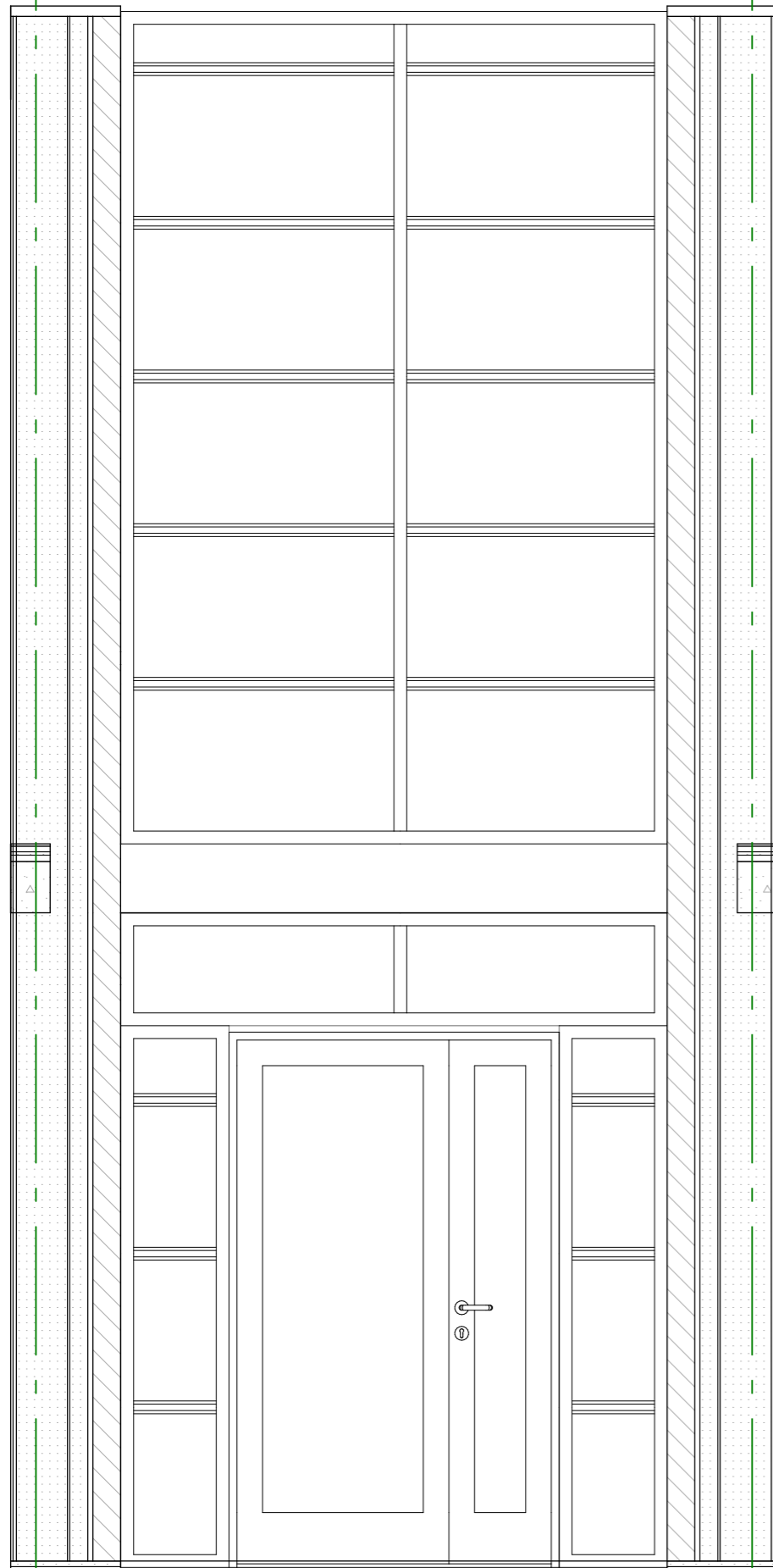
Oppriss syd 1:25
