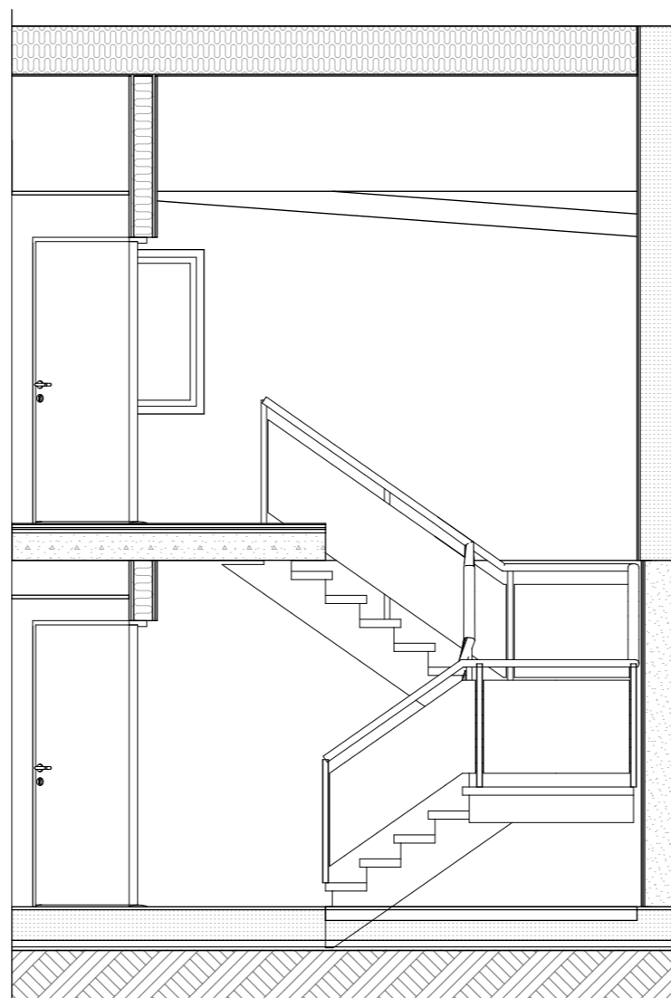
VSD02 Trapp 1:50
