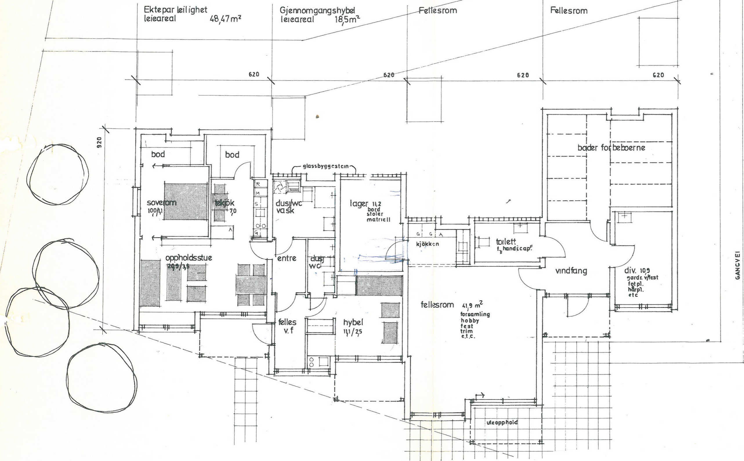
TEGNING AV GRUNNMUR SOM SKAL RIVES ETTER BRANN.
