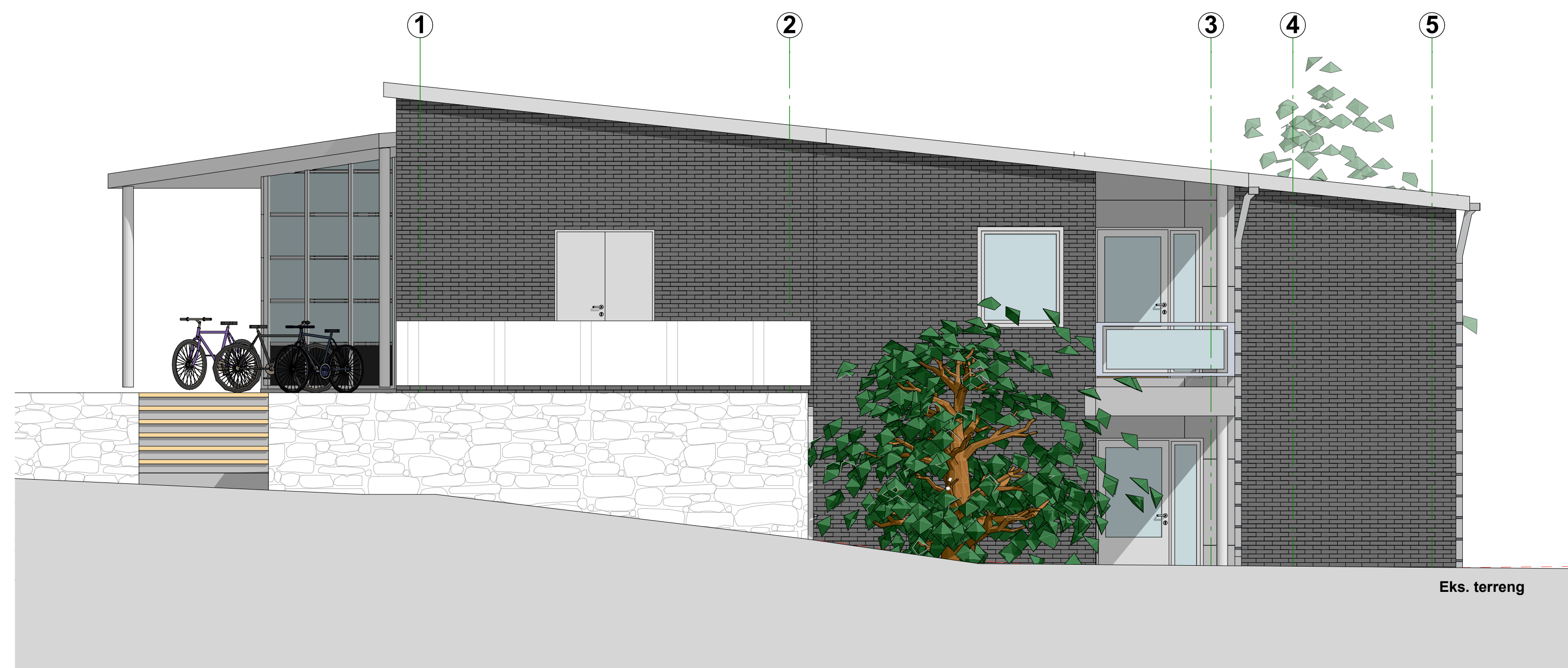
Fasade mot vest 1:50
