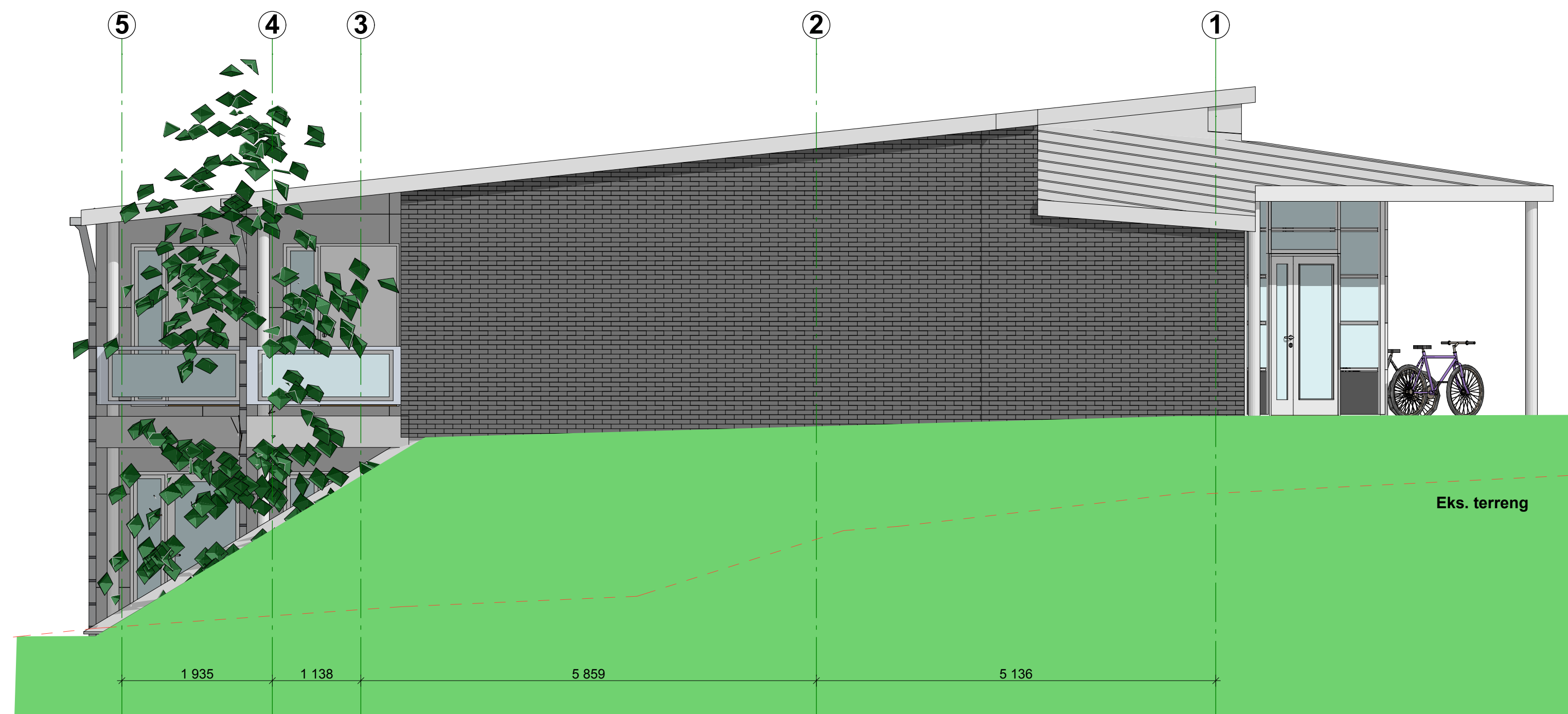
Fasade mot øst 1:50
