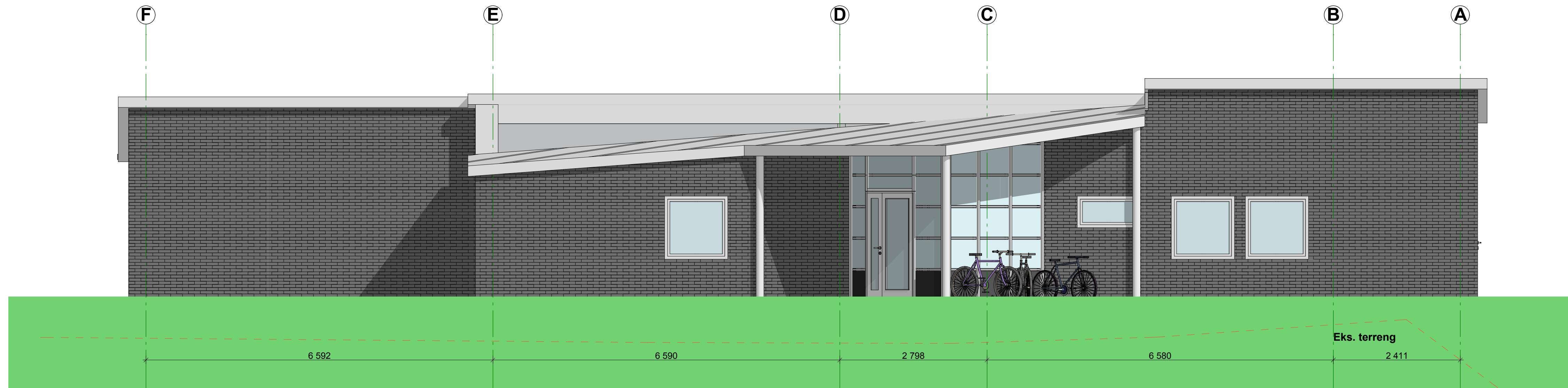
Fasade mot nord 1:50
