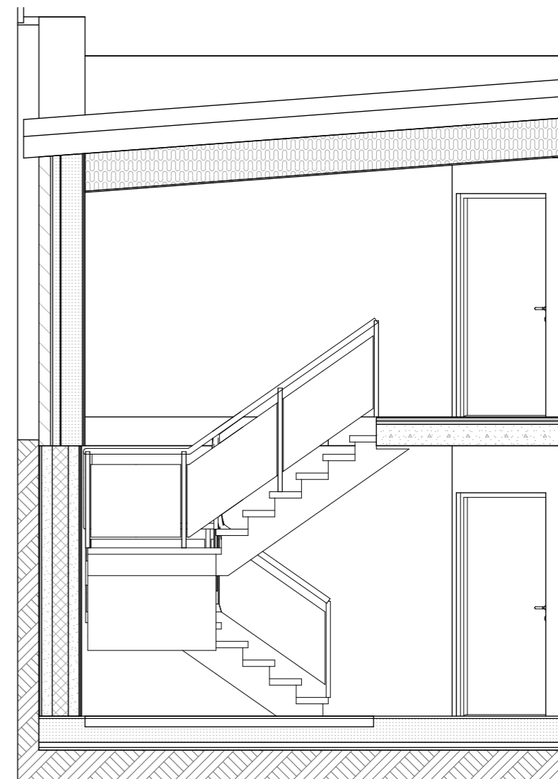
VSD03 Trapp 1:50
