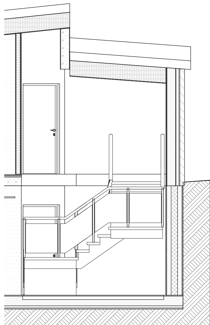
VSD01 Trapp 1:50
