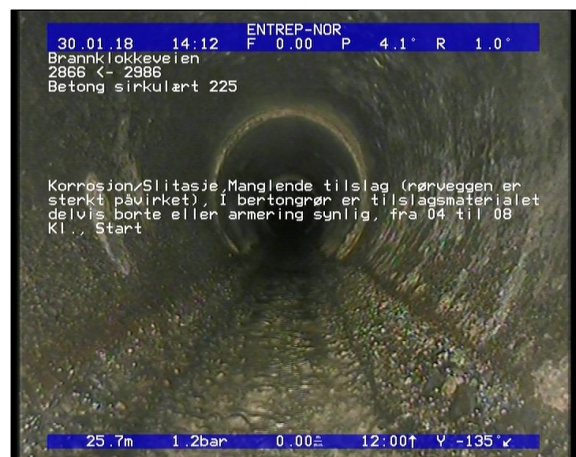
Foto: Korrosjon/Slitasje, Manglende tilslag (rørveggen er sterkt påvirket), I bertongrør er tilslagsma.JPG 25,77m, Korrosjon/Slitasje, Manglende tilslag (rørveggen er sterkt påvirket), I bertongrør er tilslagsmaterialet delvis borte eller armering synlig, fra 04 til 08 Kl., Start
