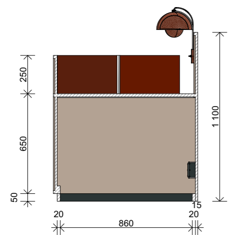
Snitt
