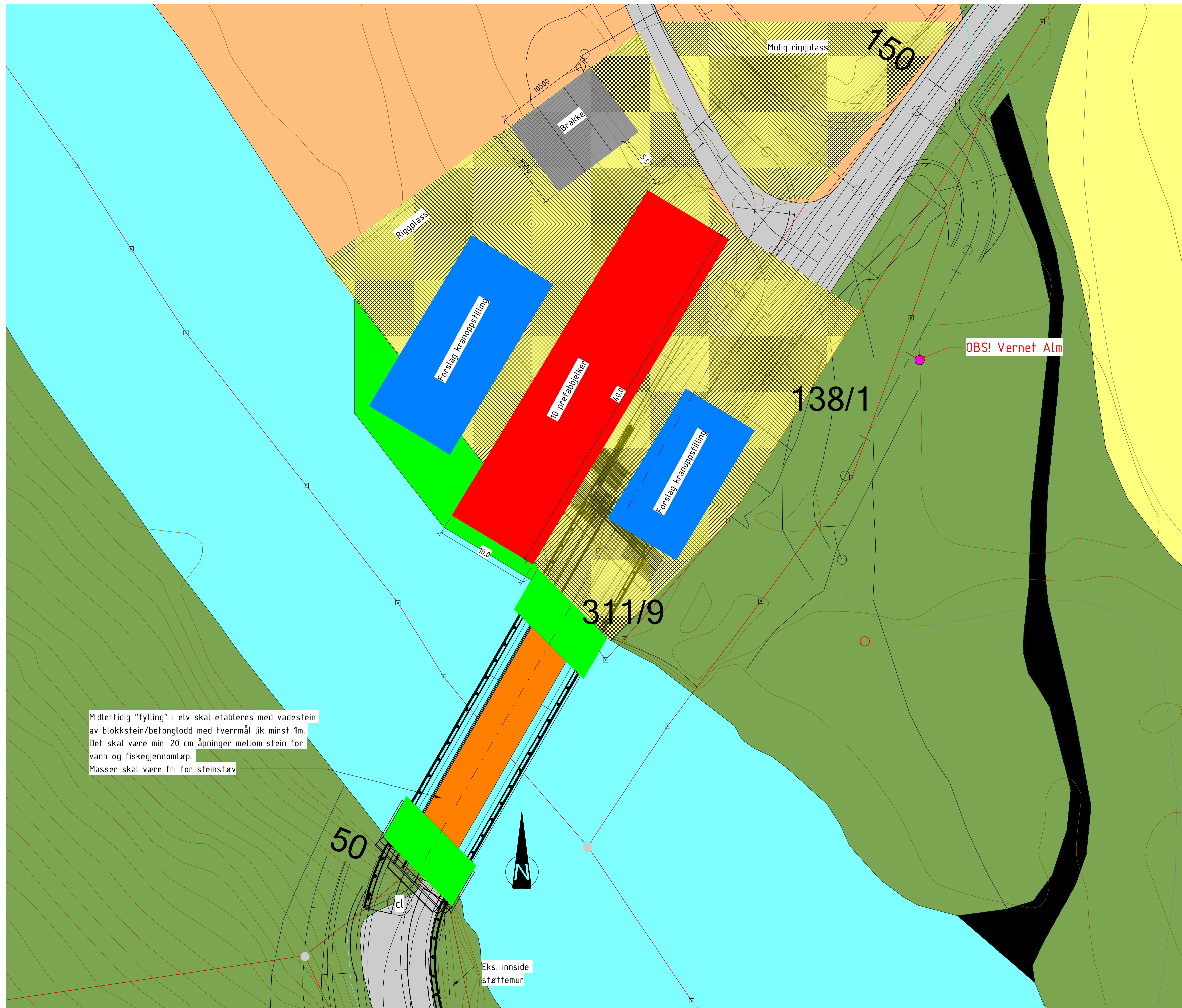
Forslag til riggplan 1 : 200
