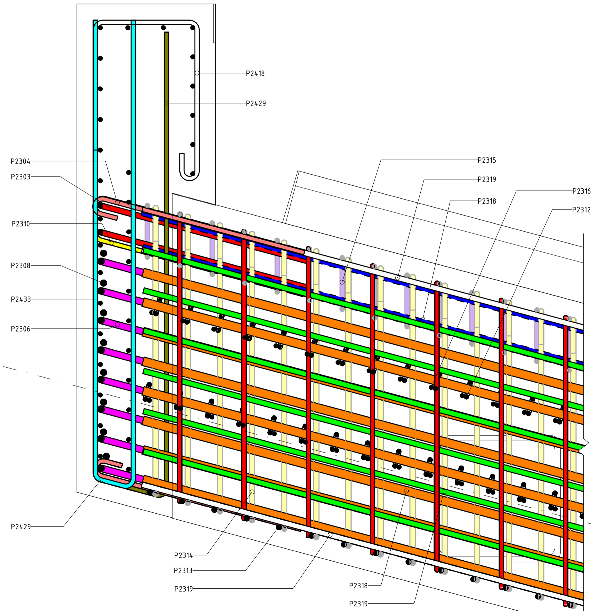
DETALJSNITT 2 - TVERRBJELKE/VINGE PLAN AKSE 2 1 : 10
