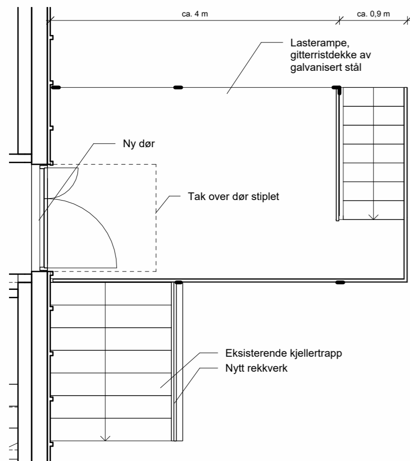
Plan varemottak 1 : 50
