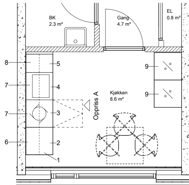
Kjøkken - plan
