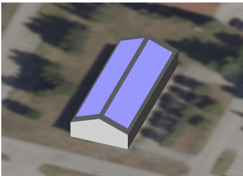
Figur 1: Illustrasjon av aktuelle flater for solcelleanlegg på bygget, sett fra sør
