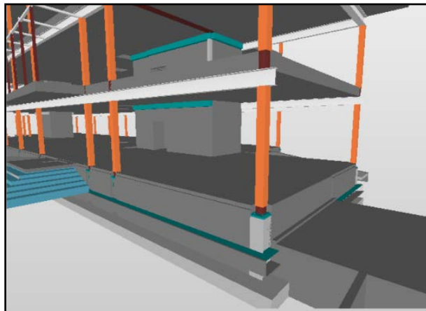
(B) Byggteknikkmodell
