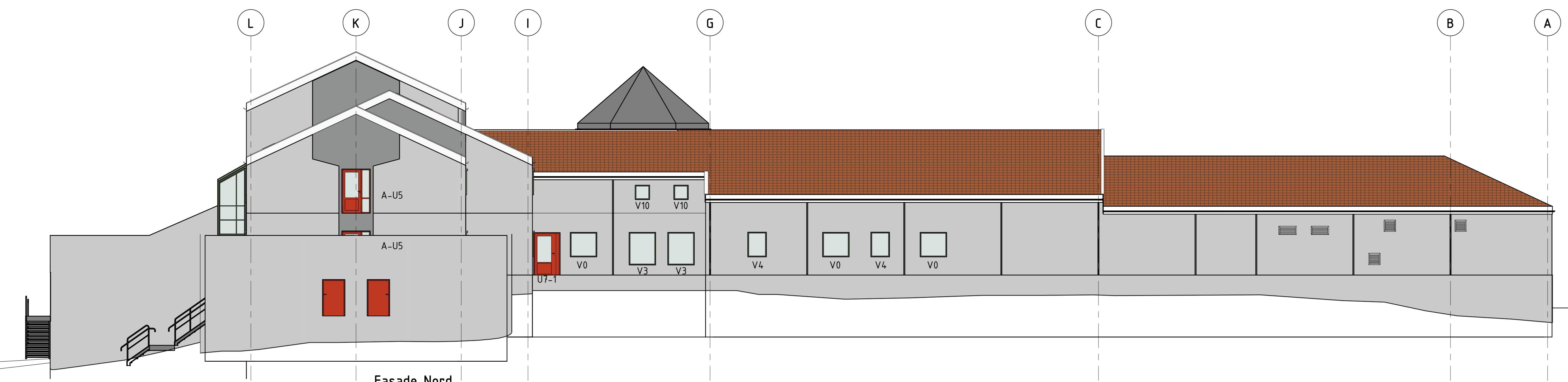
Fasade Nord 1:100
