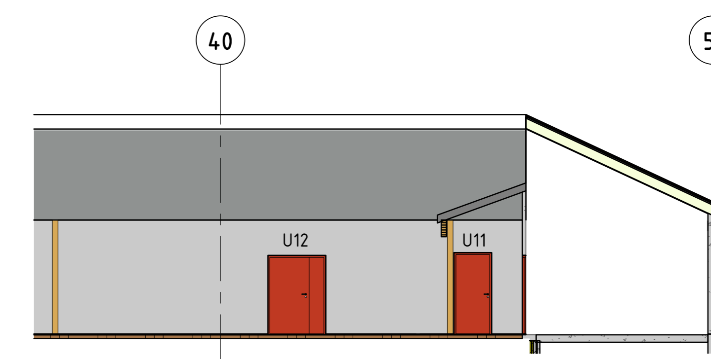
Fasade verkstedgård akse B 1:100
