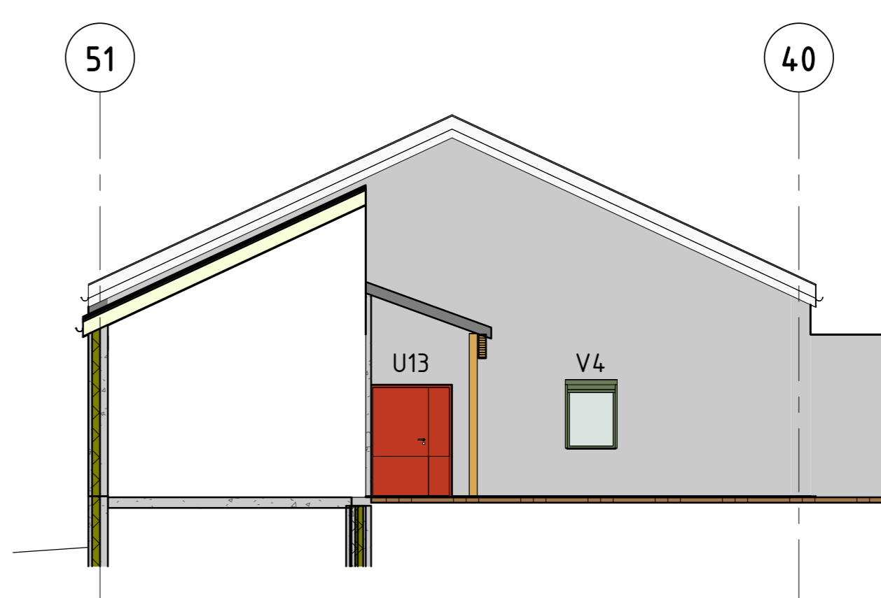
Fasade verkstedgård akse C 1:100
