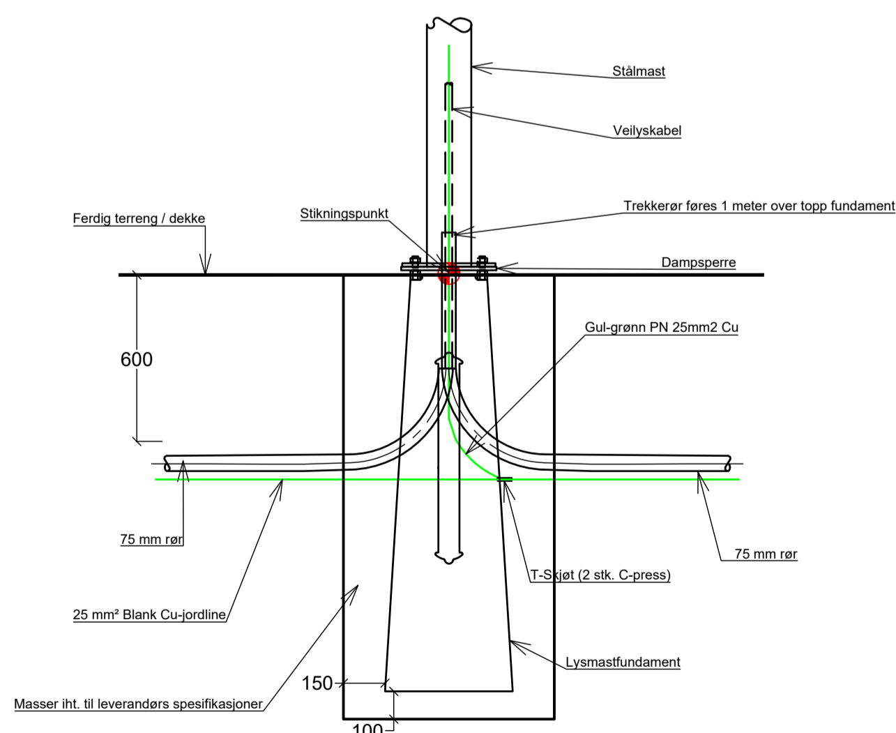
Prinsipp innføring av trekkerør i fundament
