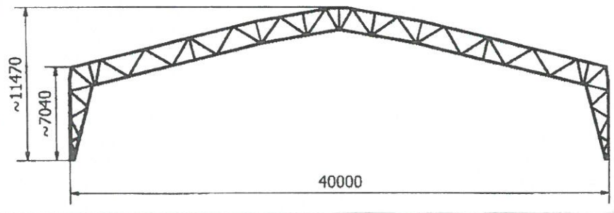
Snitt M1:250
