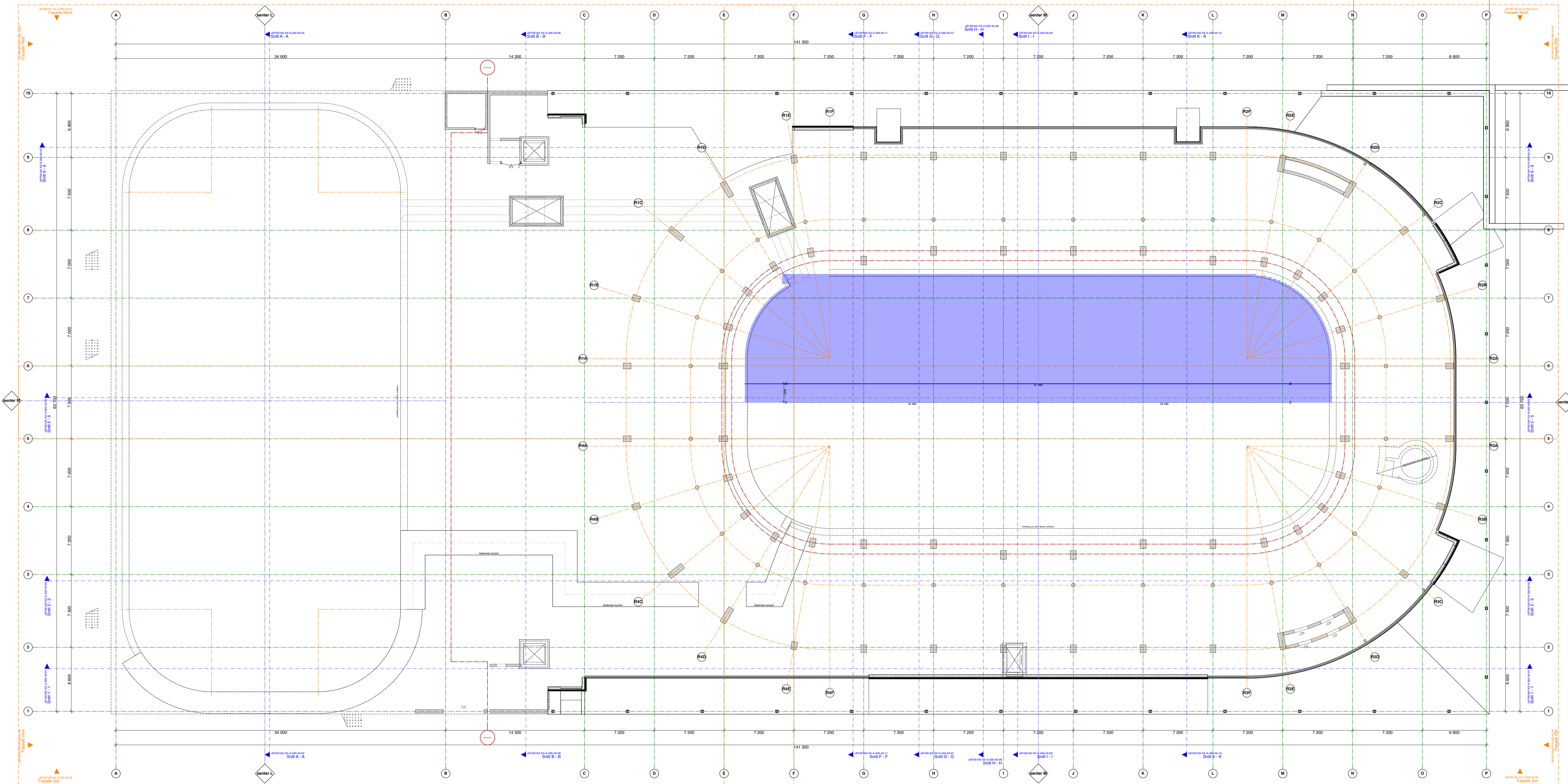
Utsnitt, plantegning: BY5619-A-H1-A-200-20-123
