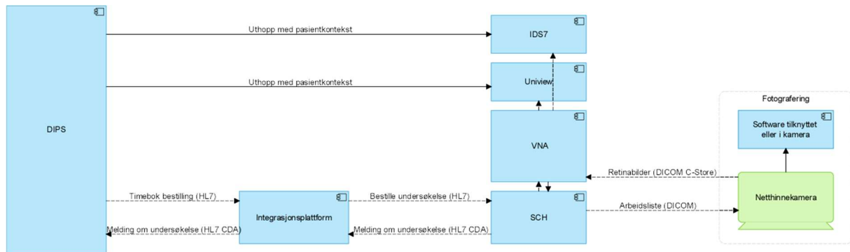
Figur 1: Plassering av netthinnekamera i sammenheng med omkringliggende systemer (Her er spesialistverktøy vist i egen boks, men dette kan også leveres som en integrert del av kamera)
