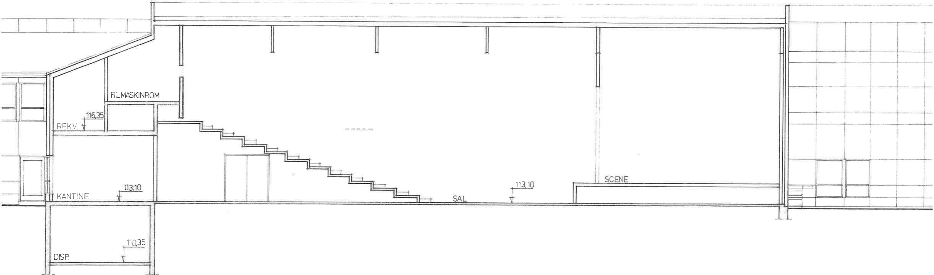
SNITT BB
