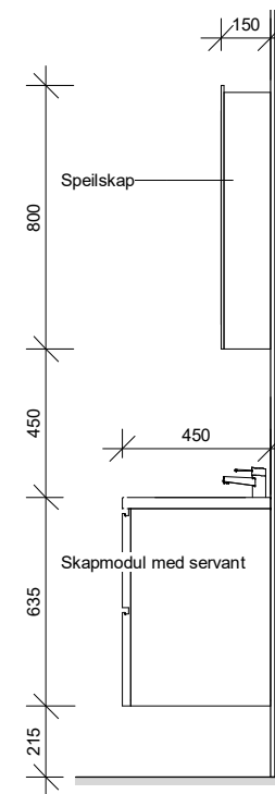
Snitt baderomsskap
