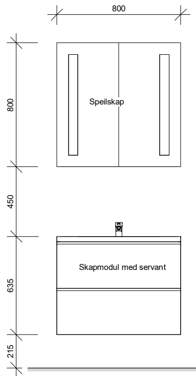
Baderomsskap 800 mm
