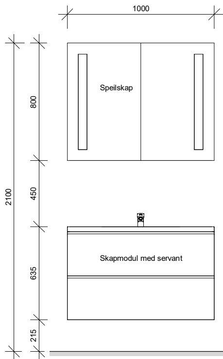
Baderomsskap 1000 mm
