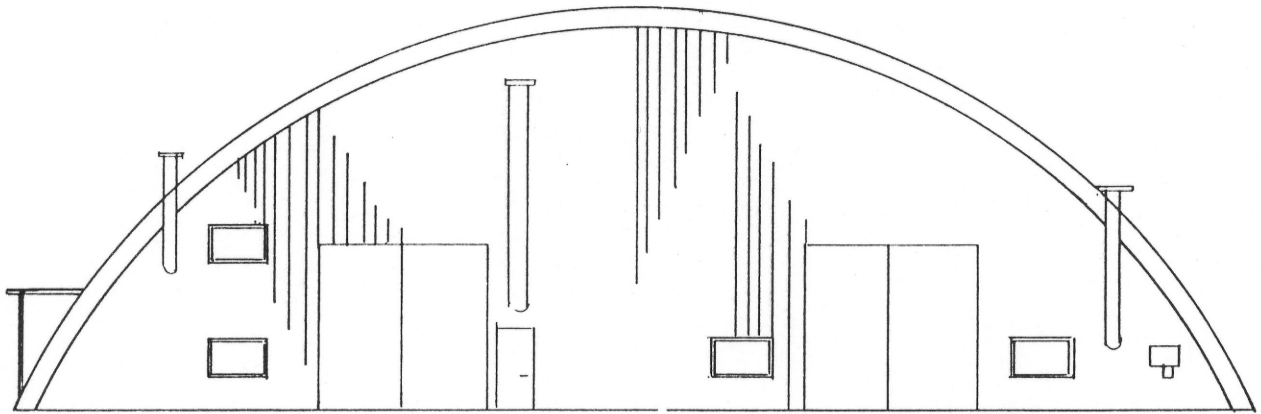
FASADE NORD-ØST
