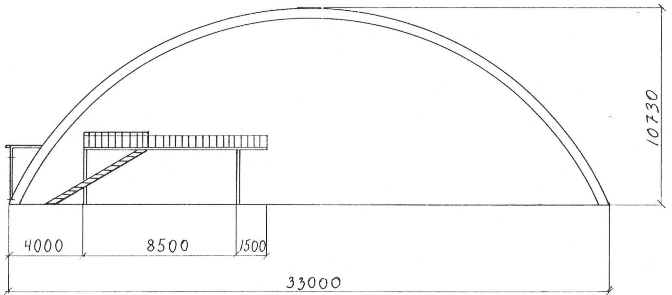
SNITT A-A
