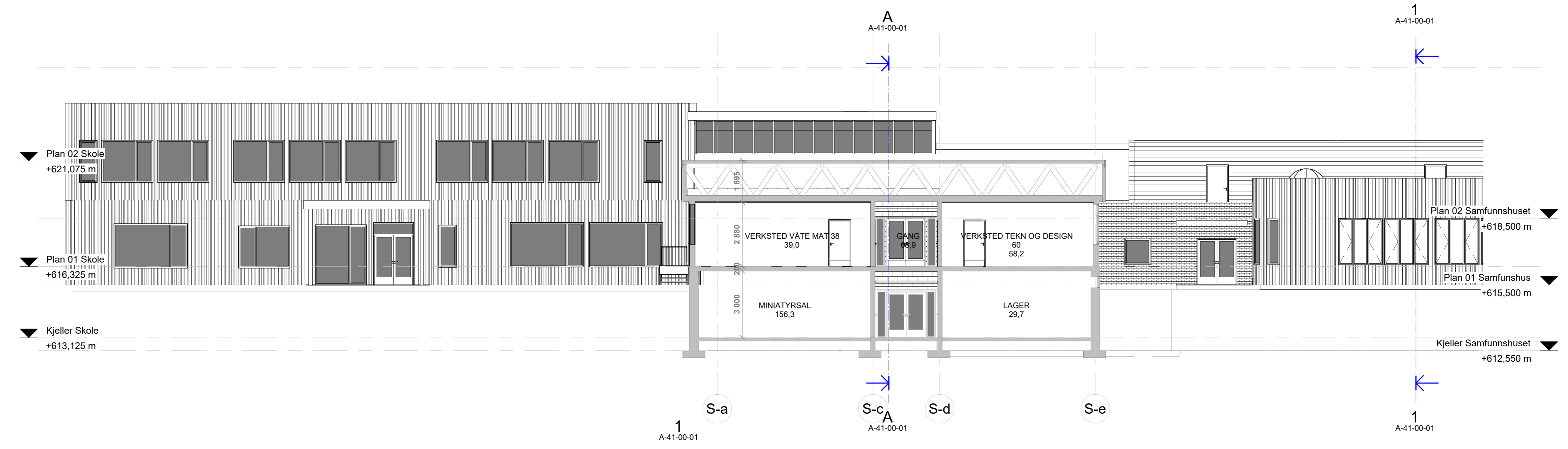
SNITT 2 - 2
