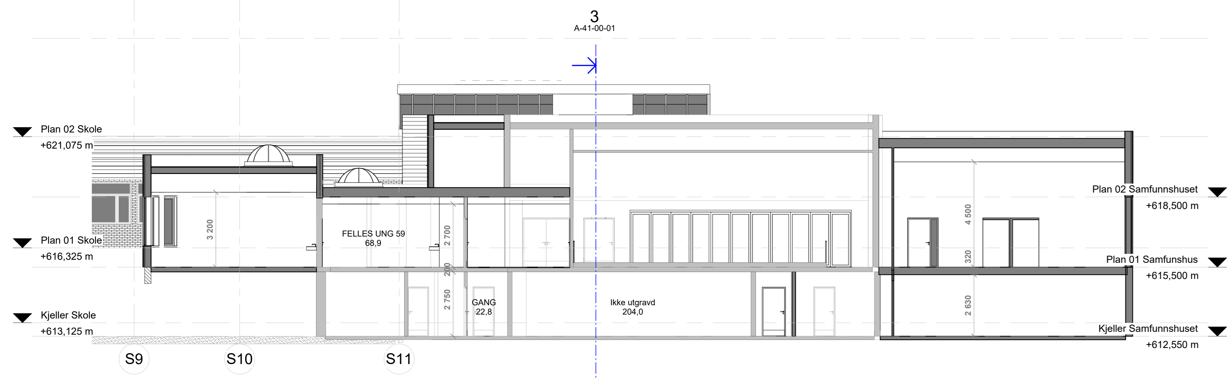
SNITT 1 - 1
