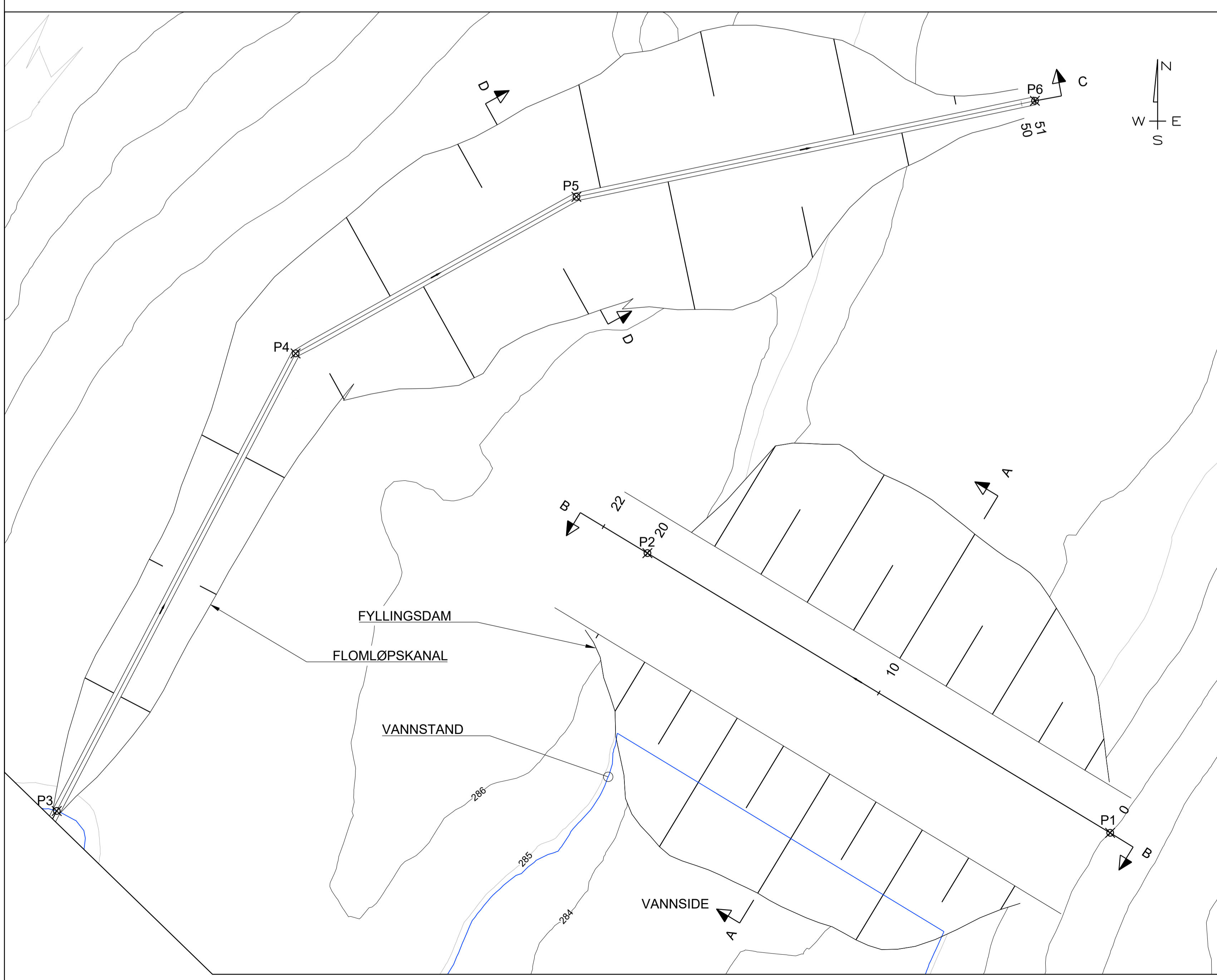
PLAN 1:100 0 1 2 5 m 1:100
