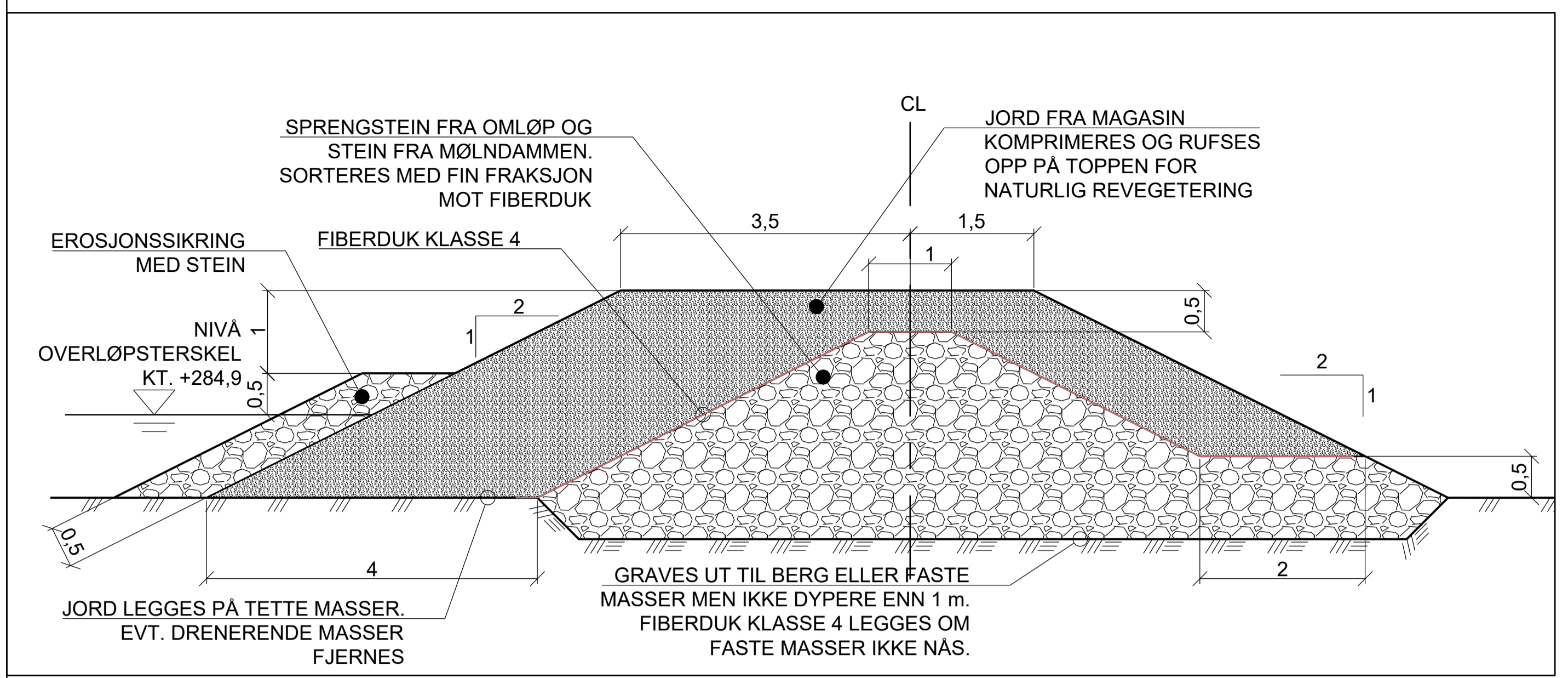
SNITT A-A 150 0 0,5 1 2,5 m 1:50
