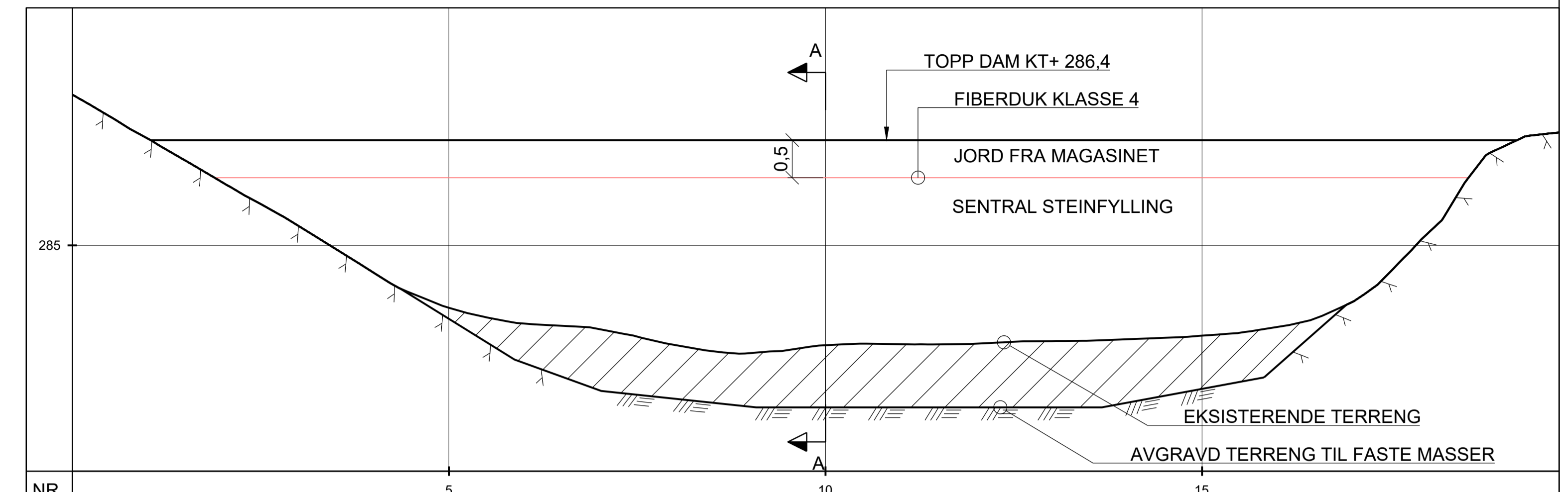
LENGDESNIITT B-B 150
