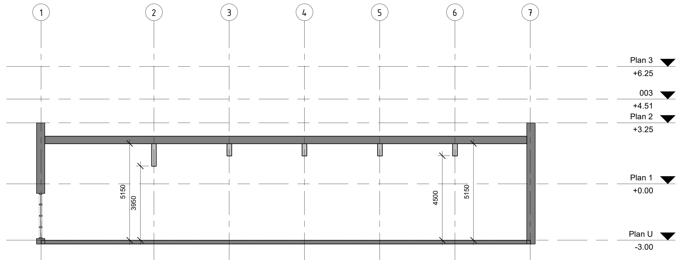
SNITT 1-EKS 1 : 100
