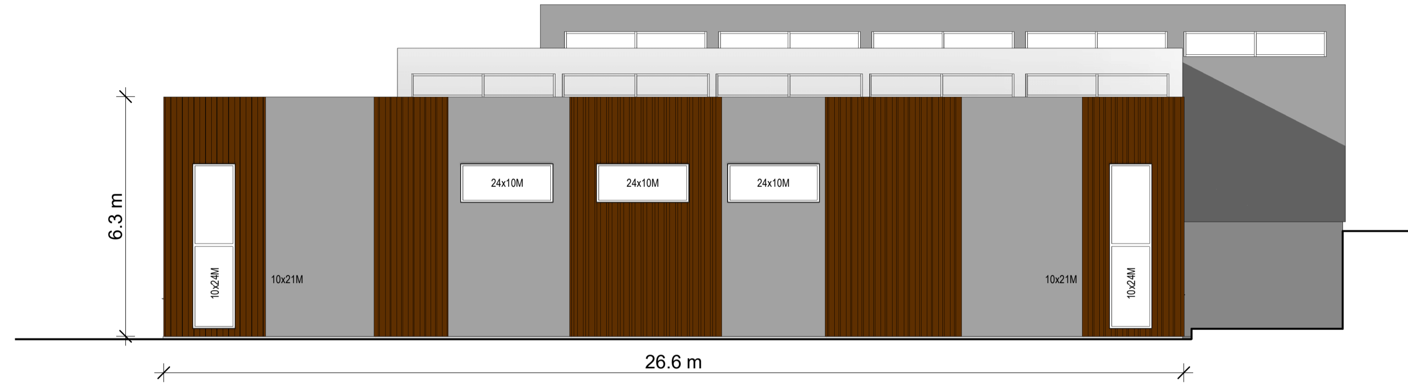
Fasade Øst NY 1 : 100
