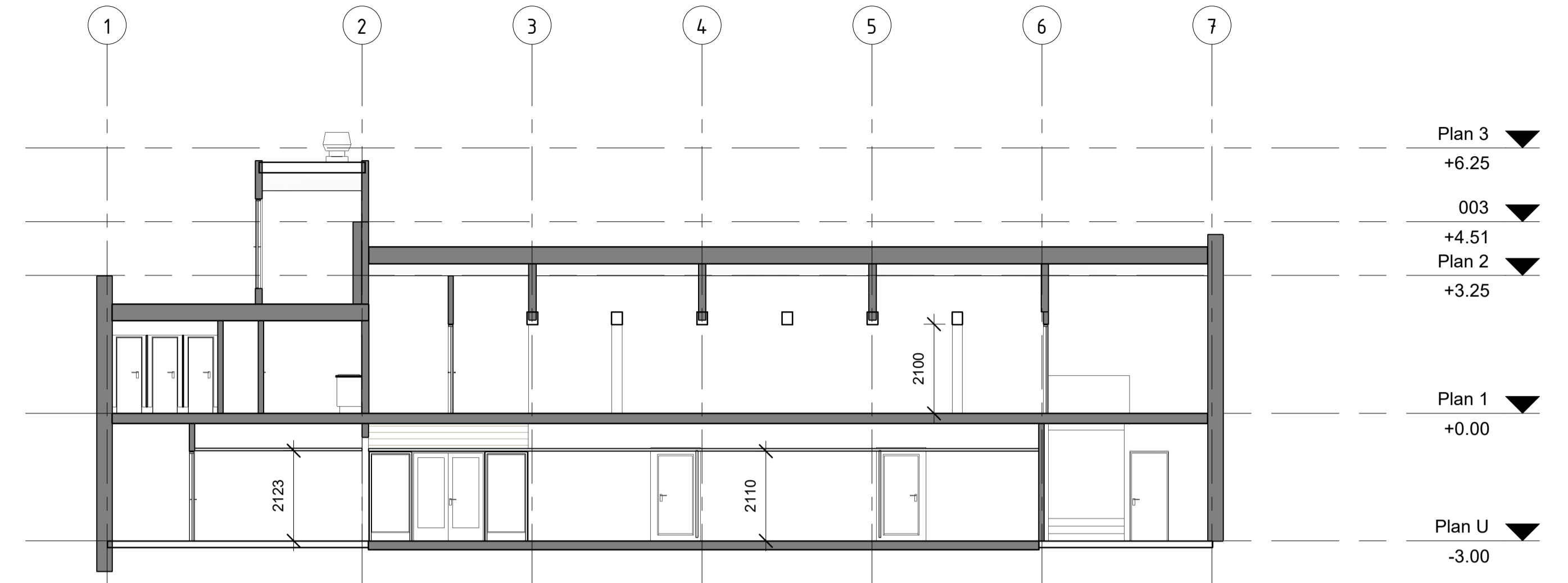
SNITT 2-EKS 1 : 100
