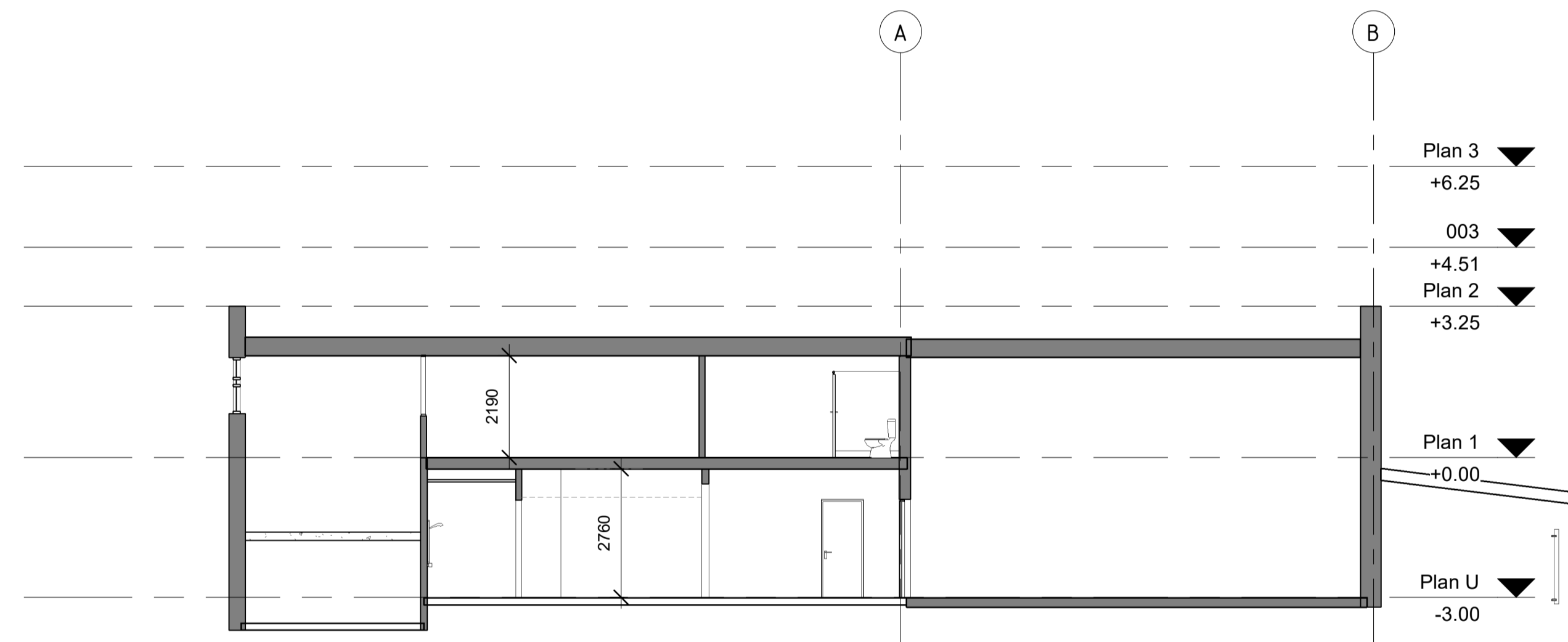
SNITT A-EKS 1 : 100
