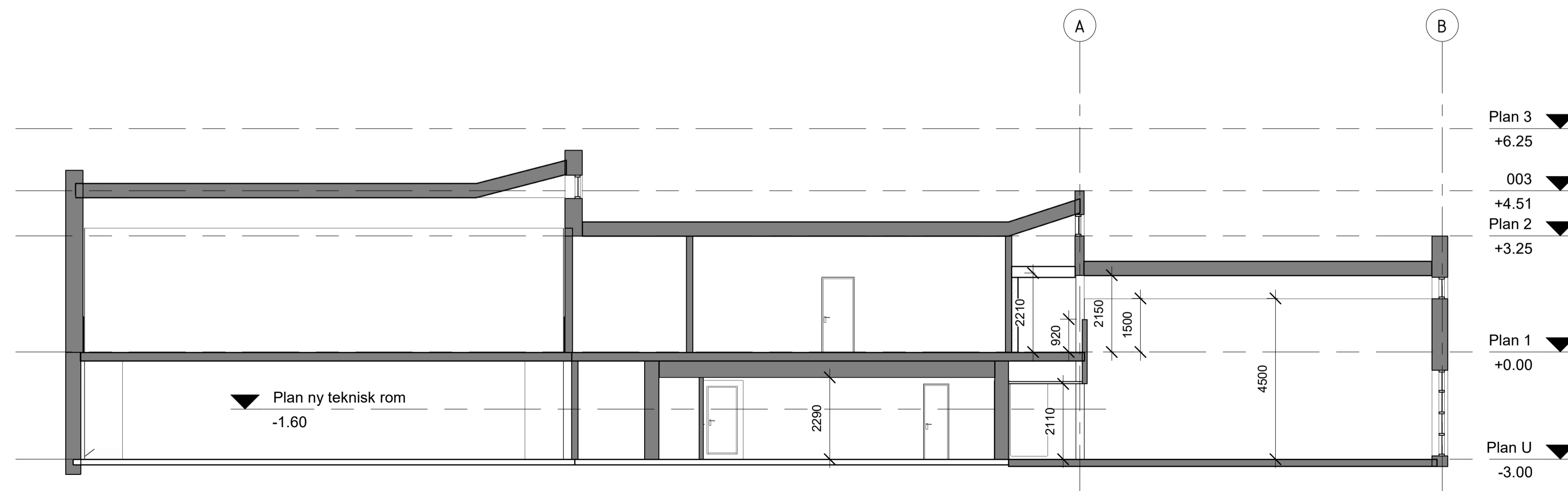
SNITT C-EKS 1 : 100
