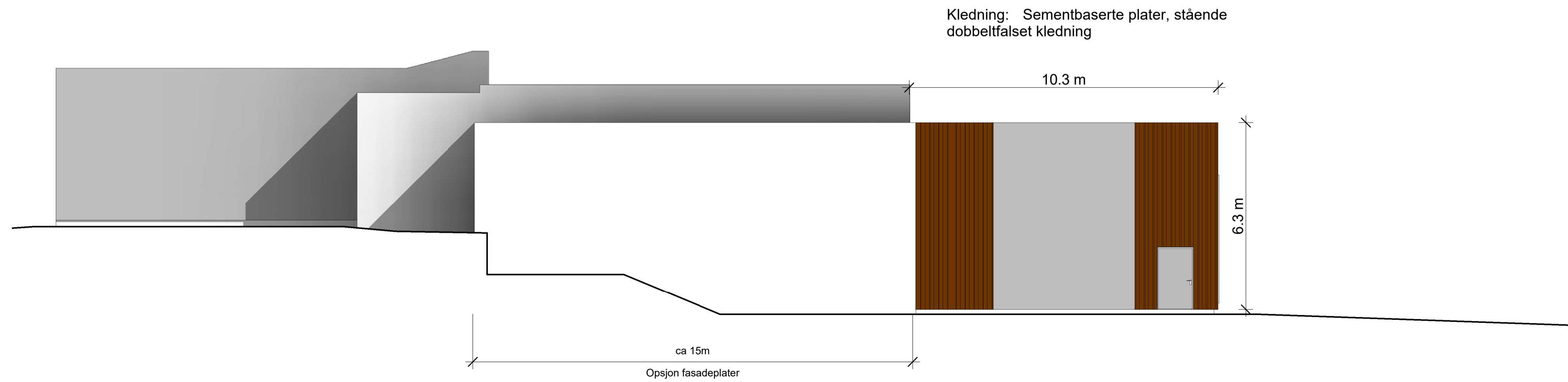
Fasade Sør NY 1 : 100
