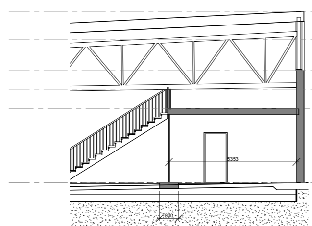
Section 1 1 : 100
