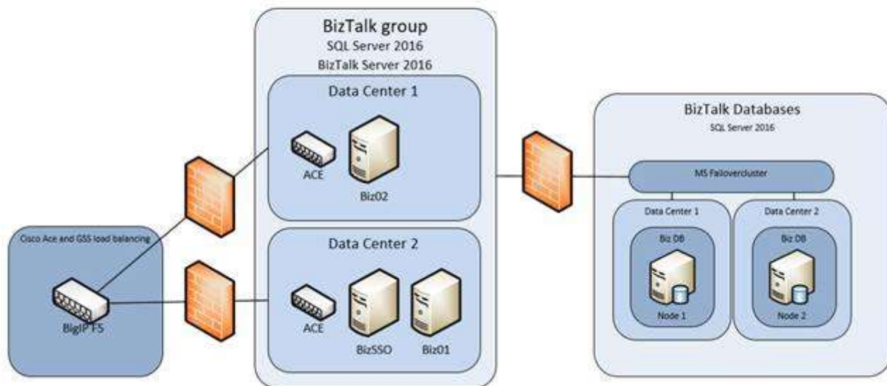
Figur 6 Overview BizTalk
