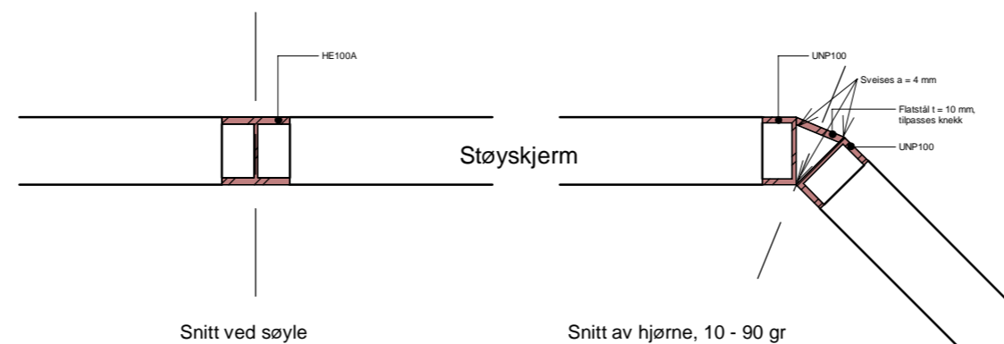
Plansnitt søyler 1 : 10
