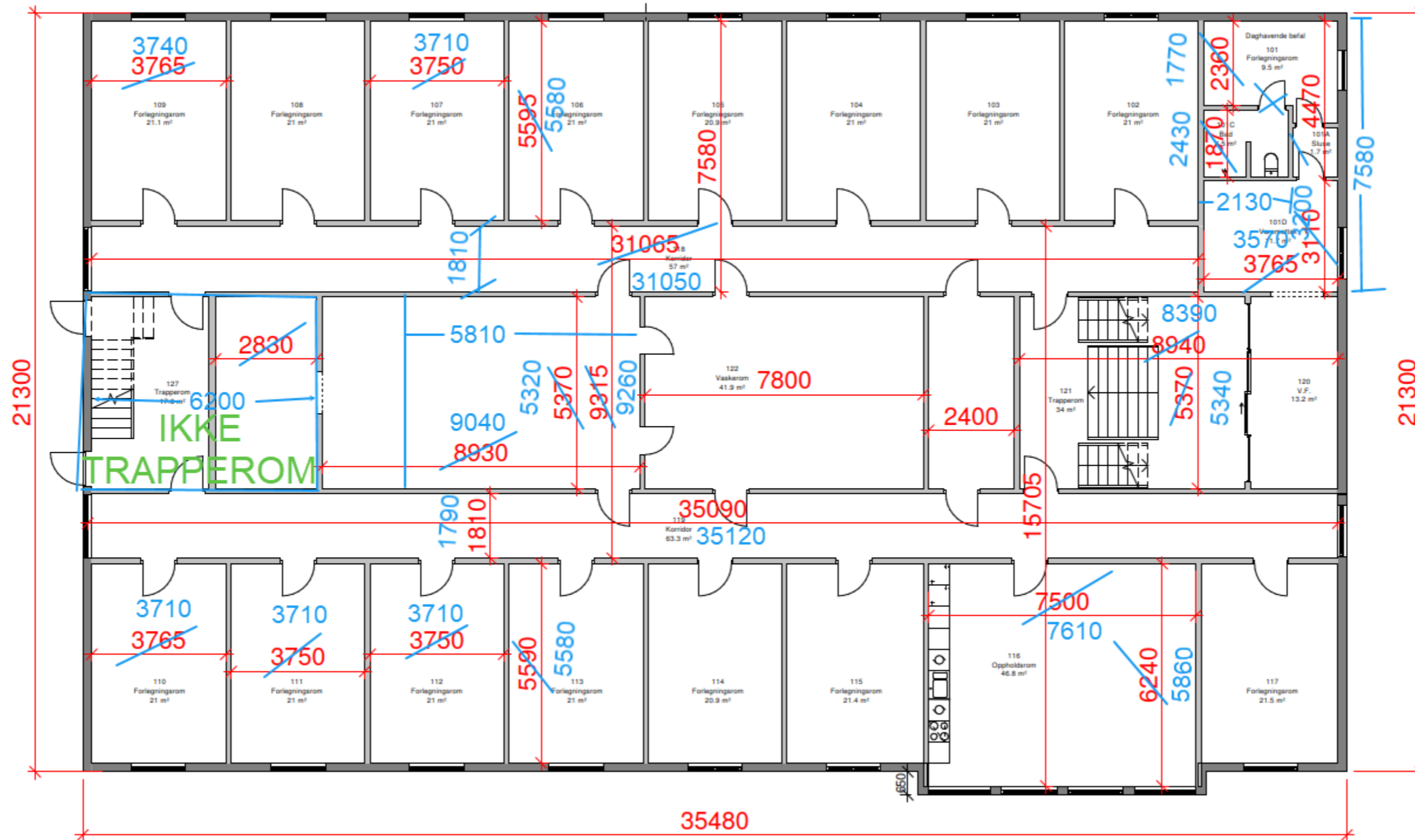
0052, Plan 1, Tegninger for målkontroll, 1:100, 20.02.2024, LPO
