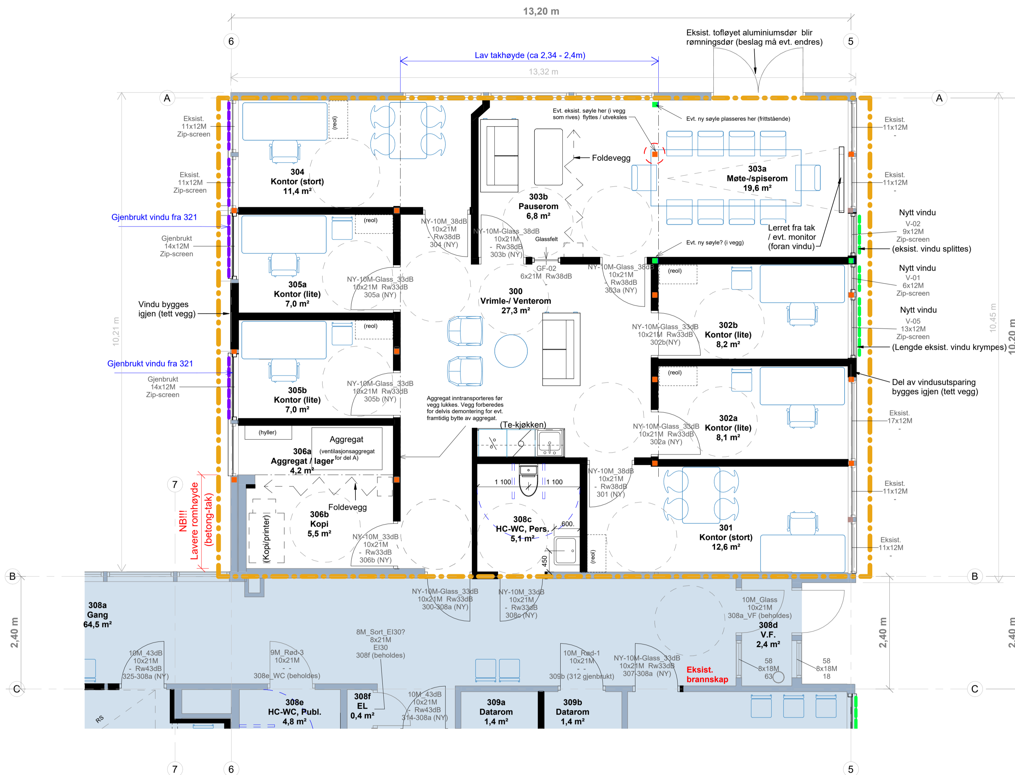
Plan 01 - Plan, etasje - Del A - (tidl. Apotek) 1 : 50
