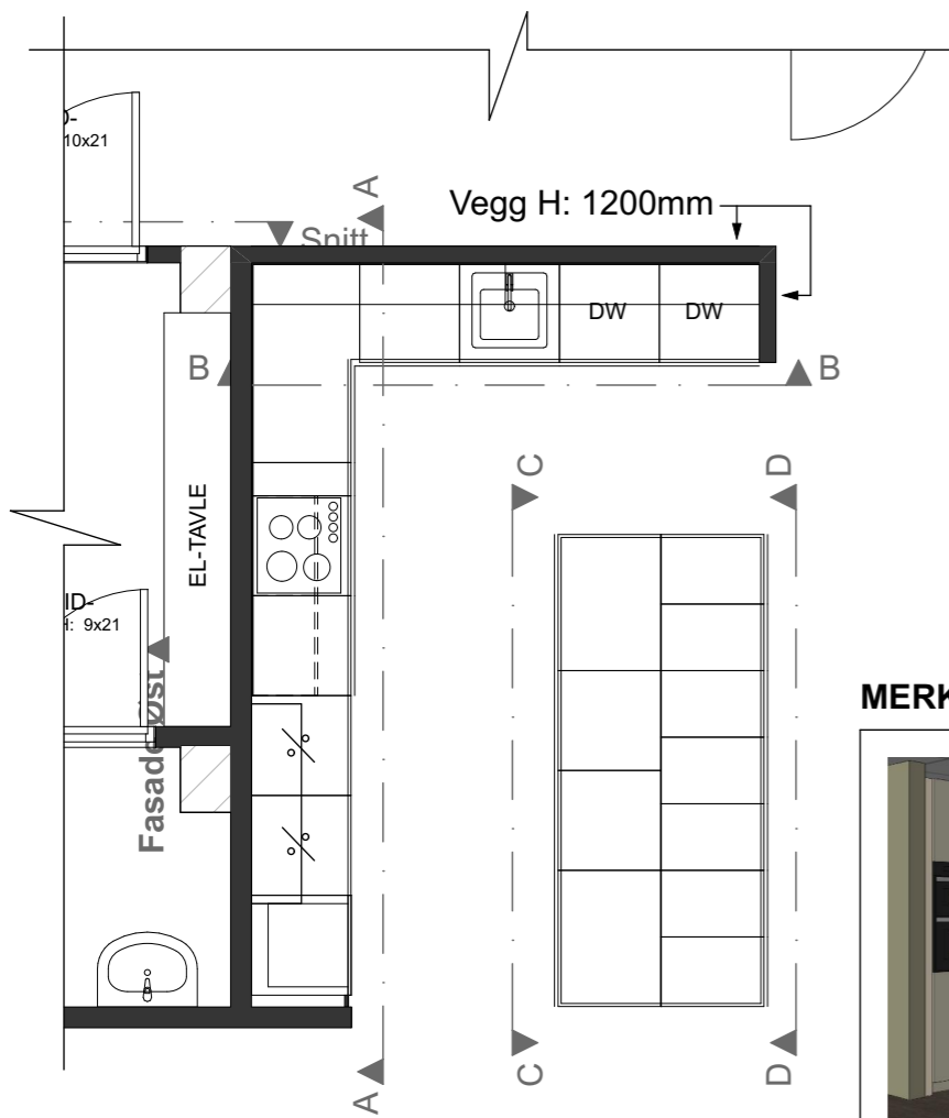
Plan Kjøkken
