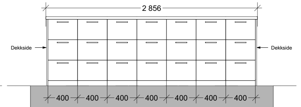
Oppriss D (kjøkkenøy)
