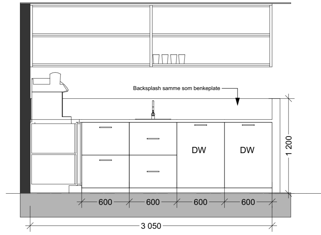
Oppriss B
