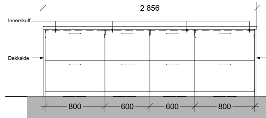
Oppriss C (kjøkkenøy)
