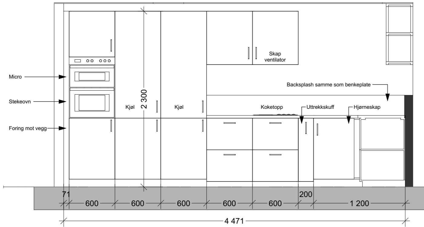
Oppriss A
